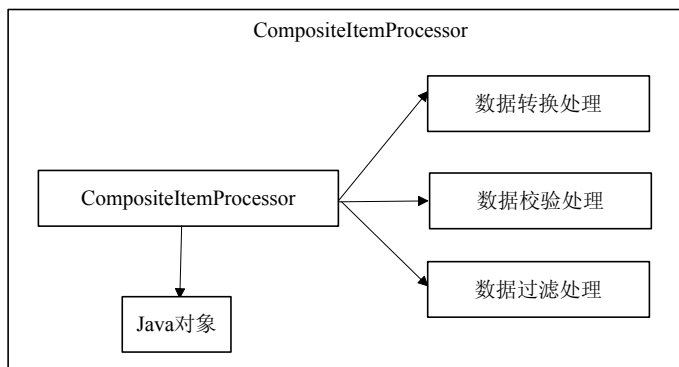
图 8-7 组合 ItemProcessor 完成的功能示意图
