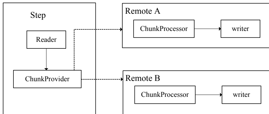
图 11-5 远程 Step 作业逻辑
