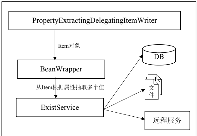
图 7-27 PropertyExtractingDelegatingItemWriter 和现有服务之间的关系
