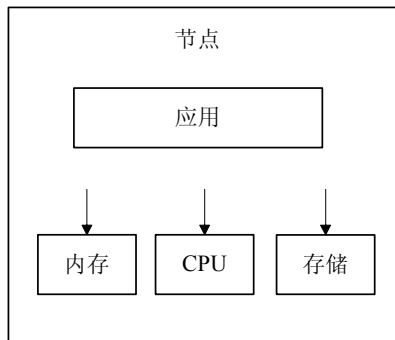
图 11-1 垂直扩展
