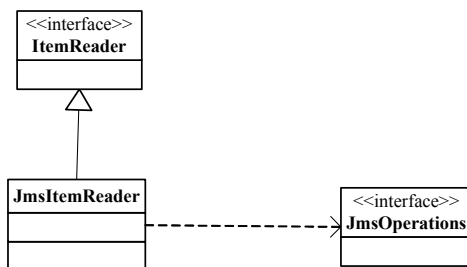
图 6-22 JmsItemReader 核心类
