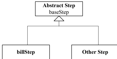
图 5-5 Step 继承
