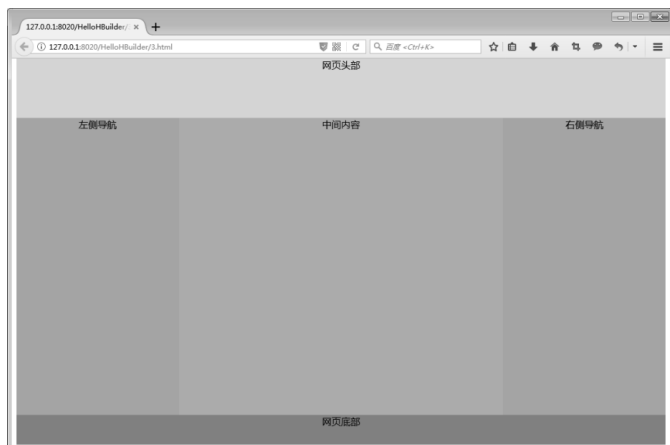
图 4-4 DIV+CSS 布局样式效果
