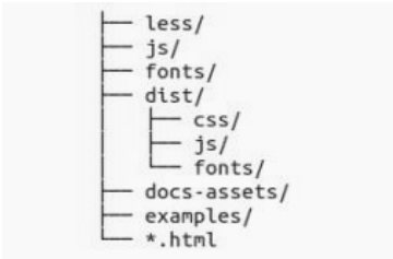
图 8-3 Bootstrap 源代码文件结构
