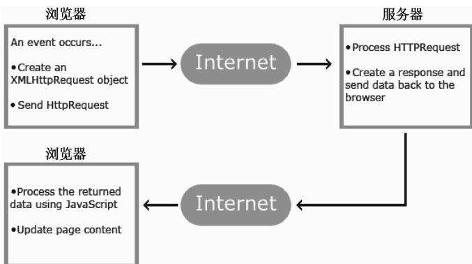
图 7-1 Ajax 工作原理图
