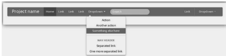
图 8-19 导航条
