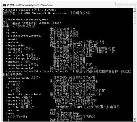
图 1-12 javac 命令信息
