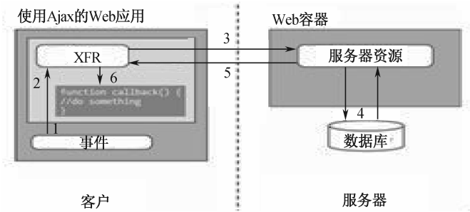
图 7-2 标准 Ajax 交互
