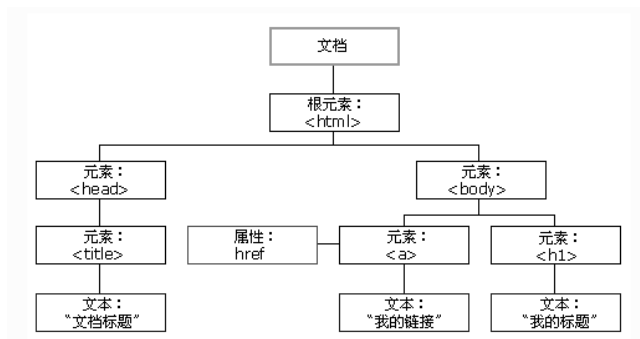
图 5-2 HTML DOM 树
