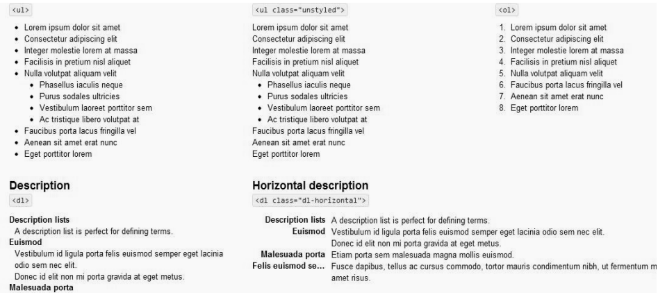
图 8-11 列表(Lists)
