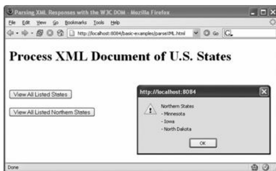
图 7-7 警告框
