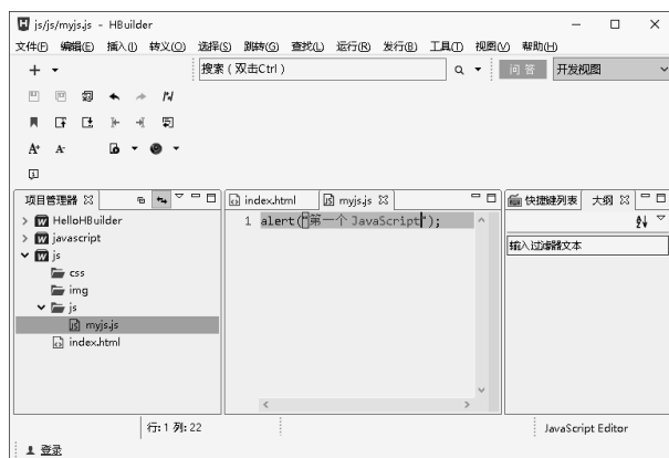
图 5-1 Hbuilder 示意图
