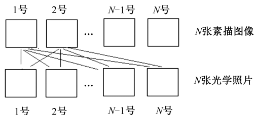
图 3.17 分组示意图
