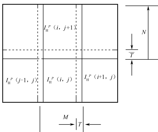
图 5.4 图像分块
