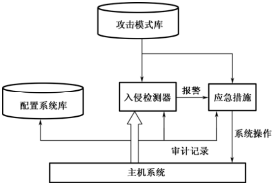
图 9.3 基于主机的 IDS 结构
