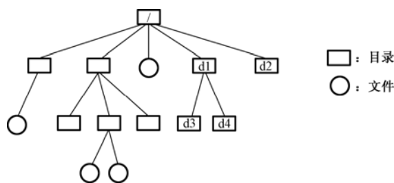
图 4.11 文件系统的树型层次结构
