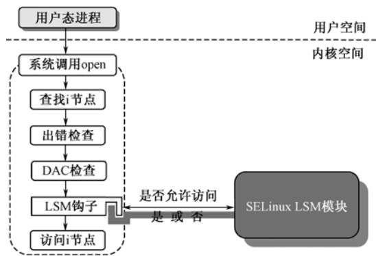
图 5.11 LSM 框架的体系结构
