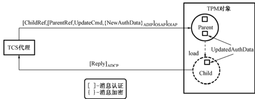
图 3.13 使用 ADCP 更新子对象的授权数据
