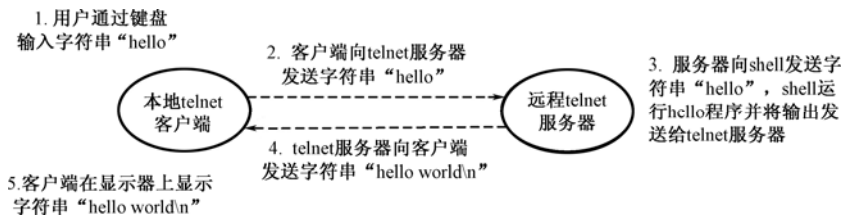
图 2.12 利用 telnet 跨越网络远程运行 hello 程序
