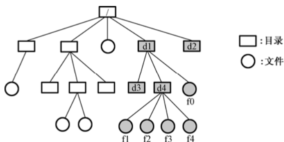
图 4.13 顶点为/d1 的子目录安装到加密安装点/d1 上
