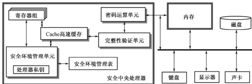
图 8.11 安全中央处理器及系统结构原理
