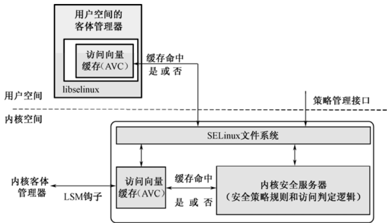
图 5.13 基于内核安全服务器的用户空间客体管理器
