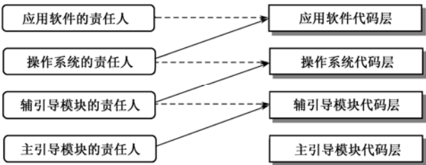
图 8.10 代码安装或更新的验证
