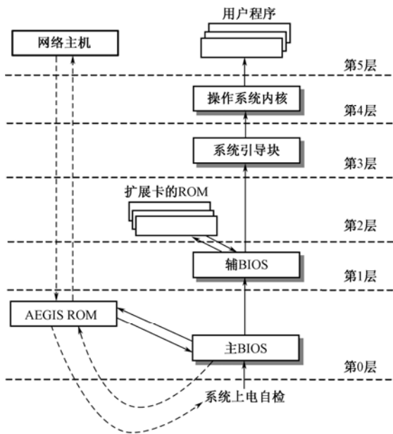
图 8.6 AEGIS 模型的安全引导过程
