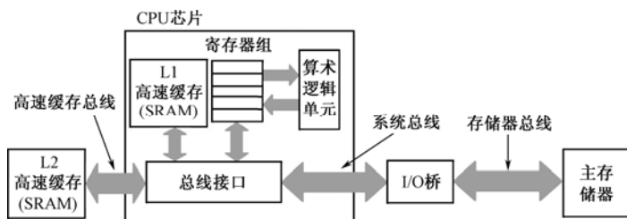
图 2.5 高速缓冲存储器
