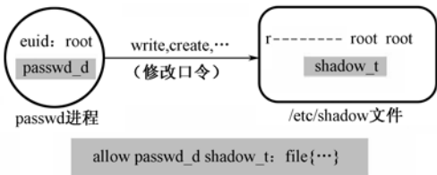
图 5.3 用 SETE 模型控制 passwd 进程
