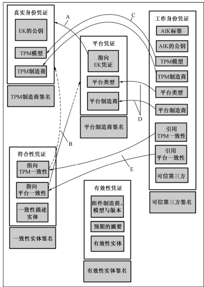
图 3.5 可信计算平台中的凭证
