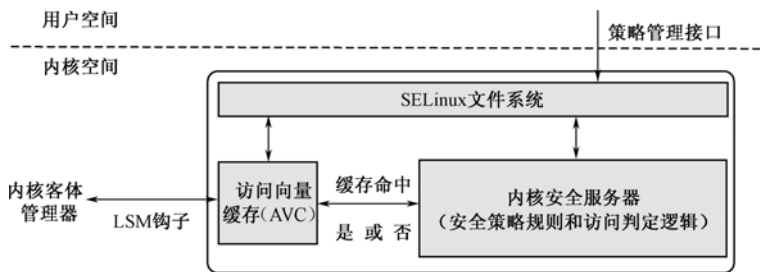
图 5.12 SELinux 的 LSM 模块的体系结构
