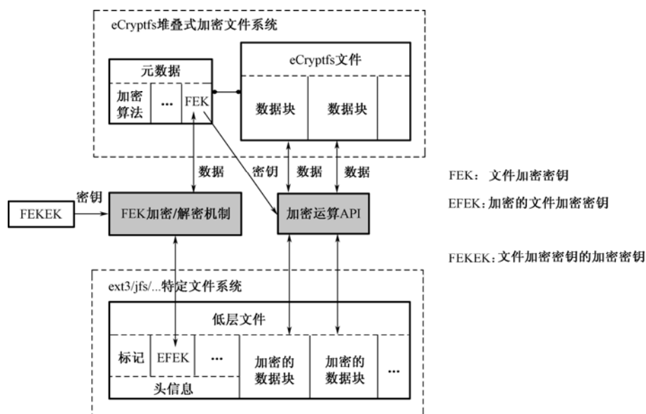
图 4.15 加密文件系统 eCryptfs 对文件的加密/解密方法
