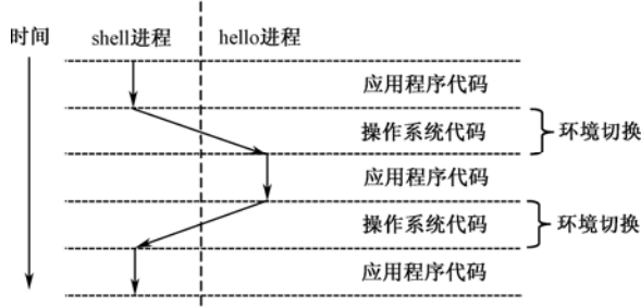
图 2.9 进程的环境切换
