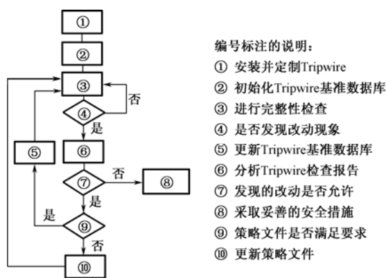
图 8.22 Tripwire 工具的应用方法
