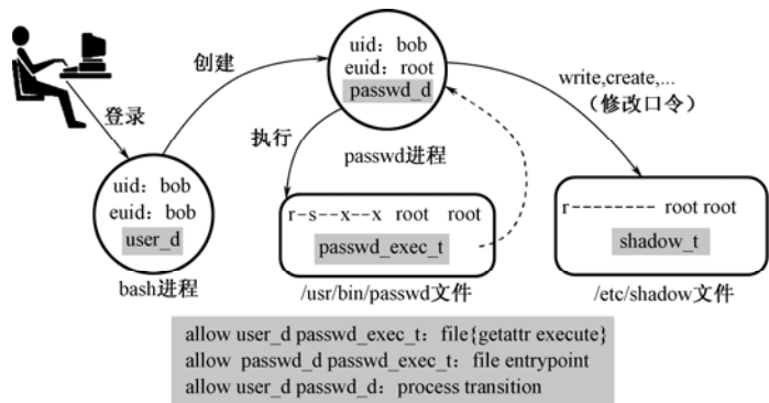
图 5.6 进程在 SELinux 中切换工作域后修改口令
