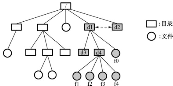
图 4.12 顶点为/d1 的子目录安装到加密安装点/d2 上
