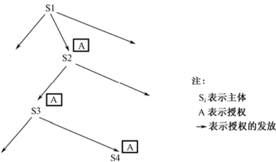
图 6.1 委托管理下的授权传递
