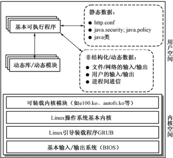
图 8.12 一个在线售书应用系统的服务器端系统组成
