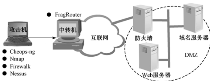
图 1.2 猎物公司网络的互联网 DMZ 和防火墙的基本结构
