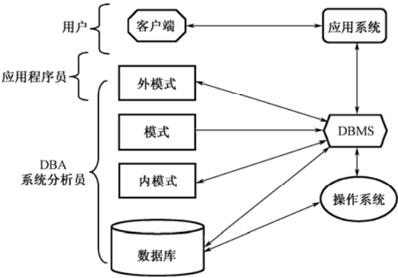
图 2.18 各种人员的数据库视图
