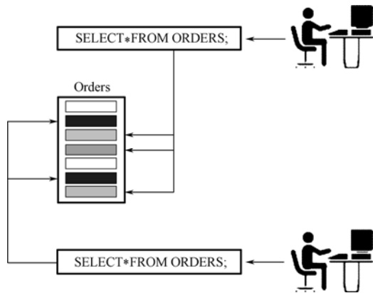
图 7.1 虚拟专用数据库思想
