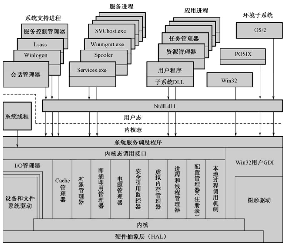
图 2.15 Windows 2000 体系结构
