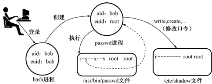
图 5.5 进程在 Linux 中改变有效身份后修改口令
