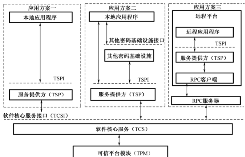
图 3.9 可信计算平台典型应用支持方案
