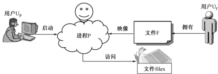
图 4.9 用户与进程和文件的关系
