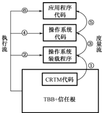
图 3.3 系统引导过程中的信任传递
