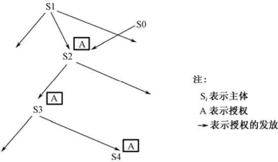
图 6.2 多方授权与授权传递
