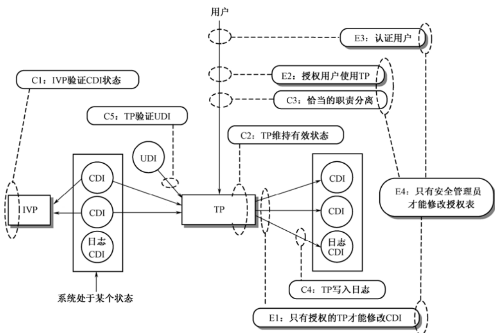
图 8.1 克-威模型的系统完整性规则
