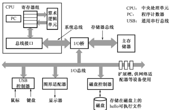
图 2.1 一个典型的计算机系统的硬件组成
