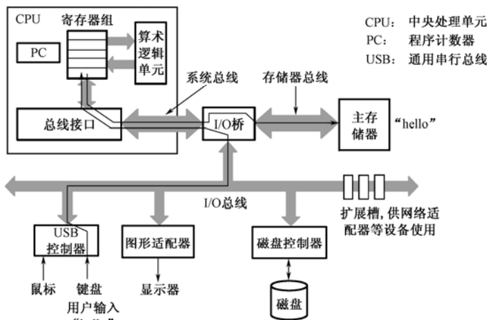
图 2.2 从键盘上读取 hello 命令
