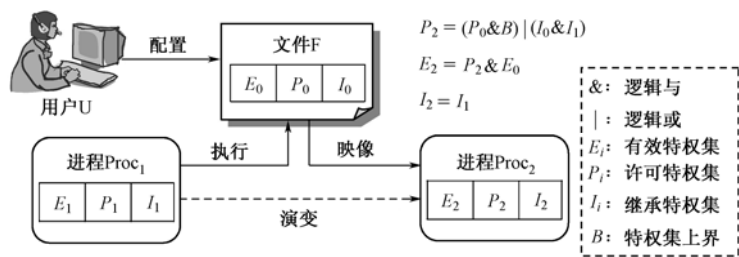
图 4.10 程序映像更新时的进程特权确定方法
