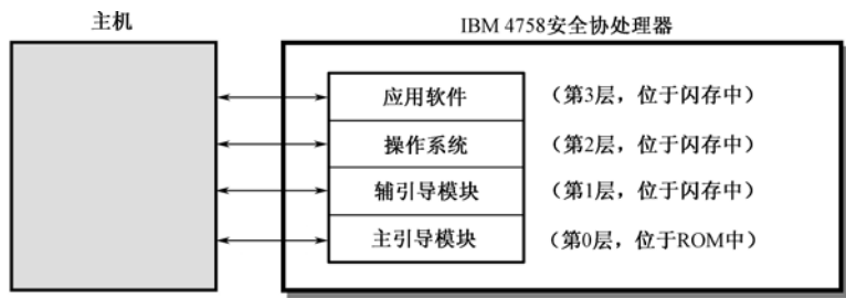
图 8.8 IBM 4758 安全协处理器的软件层次结构
