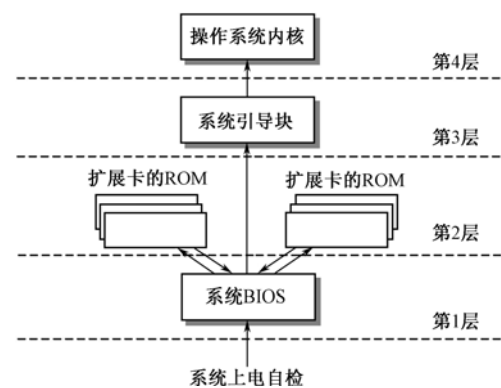
图 8.4 普通 PC 的一般引导过程
