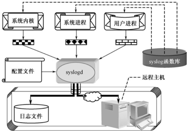
图 4.16 syslog 审计服务系统的结构
