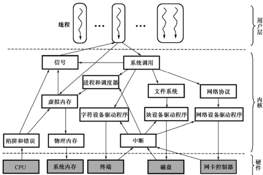
图 2.14 Linux 操作系统内核的主要组件
