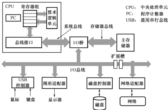
图 2.11 网络也是一种 I/O 设备
