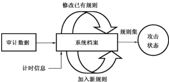
图 9.5 滥用检测系统
