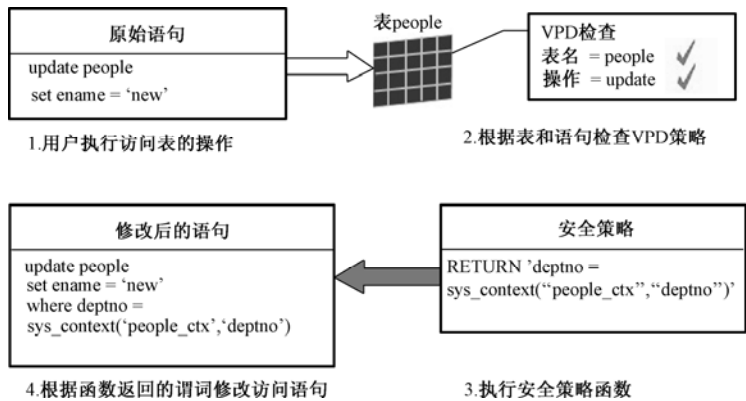
图 7.2 VPD 机制的访问控制过程
