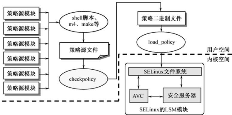
图 5.16 SELinux 安全策略的构造与装载方法
