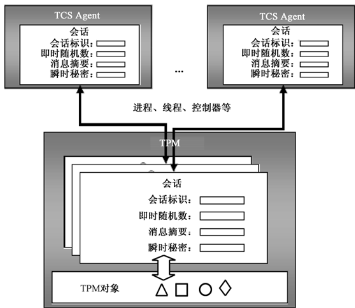
图 3.10 命令授权验证会话
