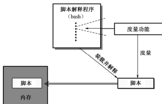
图 8.18 可执行脚本的装载和完整性度量
