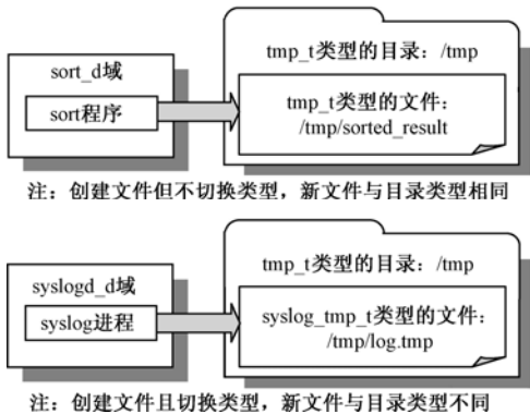
图 5.10 文件创建与切换判定
