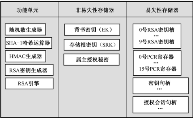
图 3.14 程序员视角的 TPM 结构
