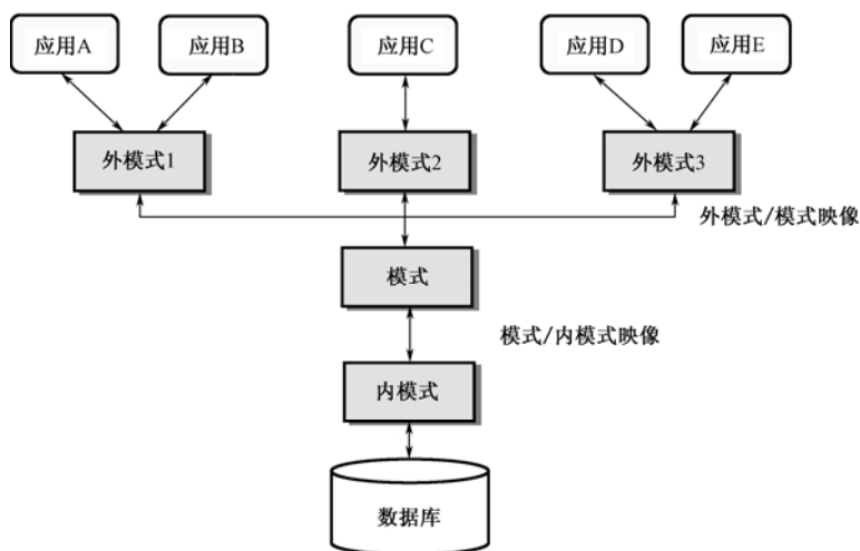
图 2.17 数据库系统的三级模式结构
