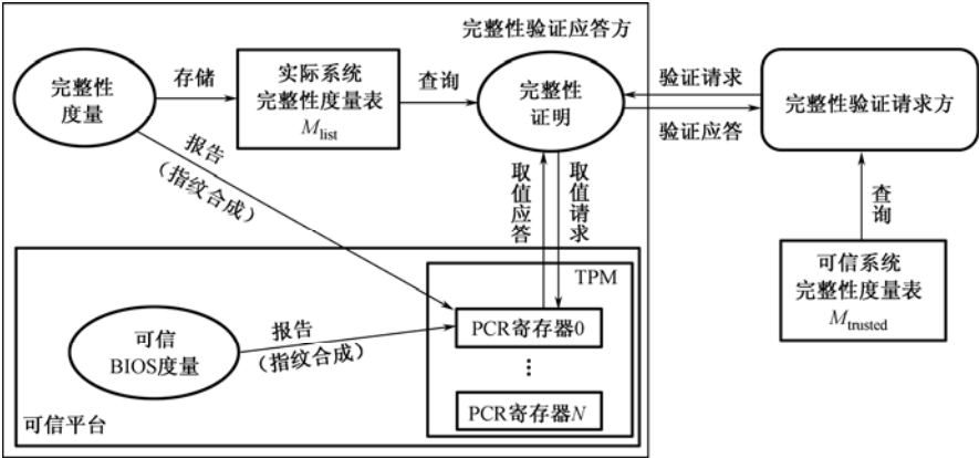
图 8.14 IMA 模型完整性度量框架
