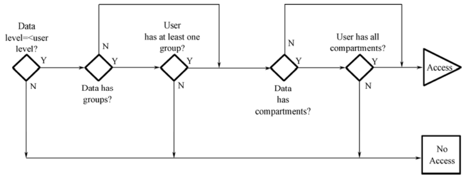
图 7.4 基于标签的读访问的判定过程
