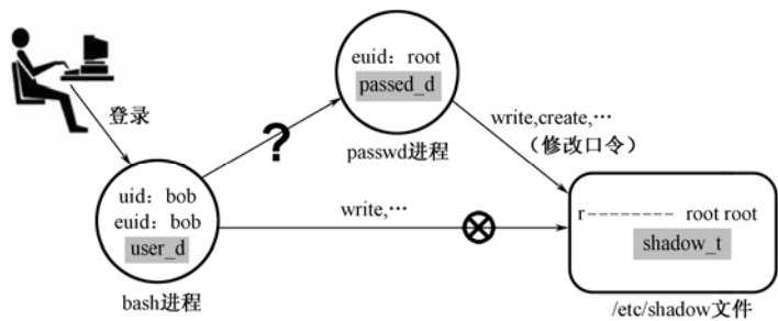
图 5.4 用户登录后欲修改口令的过程
