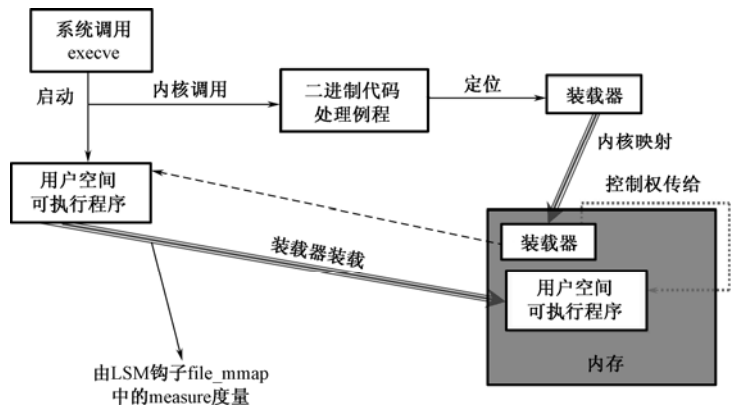
图 8.16 可执行程序的装载和完整性度量
