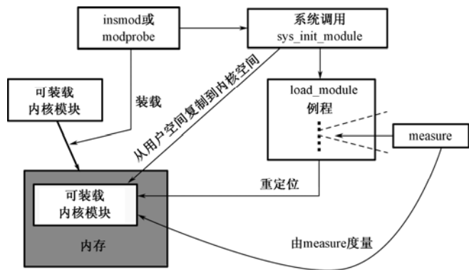
图 8.15 可装载内核模块的装载和完整性度量
