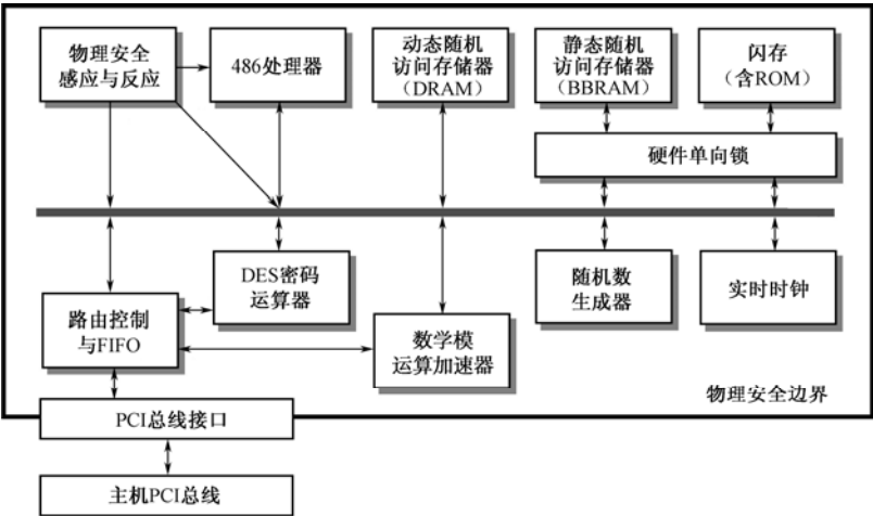
图 8.7 IBM 4758 安全协处理器的硬件组织结构
