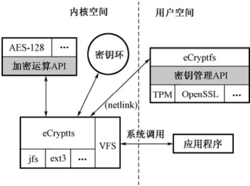
图 4.14 加密文件系统 eCryptfs 的基本结构和原理
