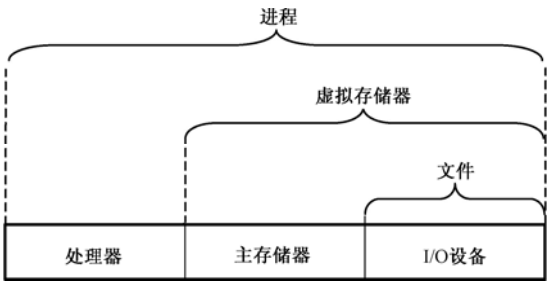
图 2.8 操作系统提供的抽象表示
