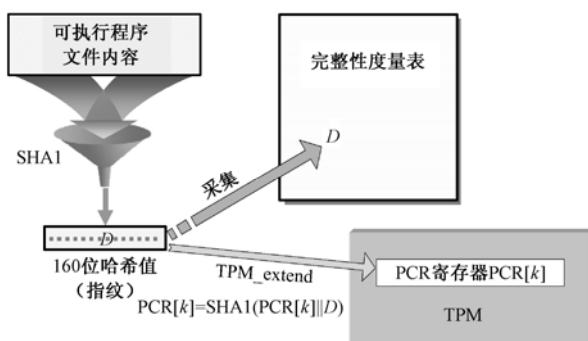
图 8.13 文件内容的完整性度量
