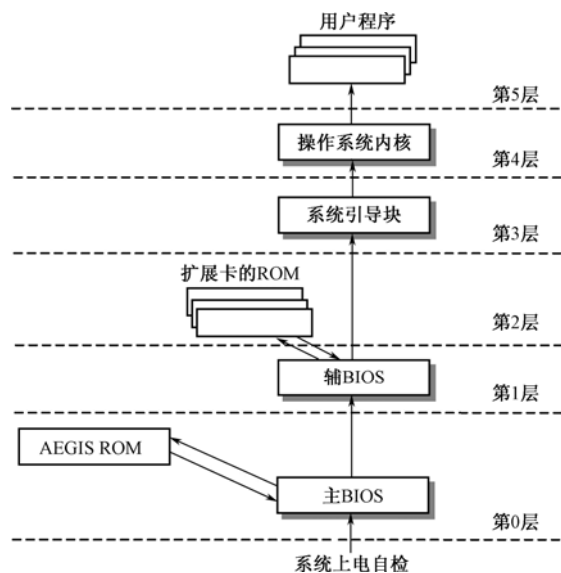
图 8.5 系统的可信引导过程
