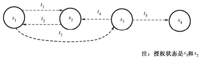
图 1.3 一个简单的有限状态自动机
