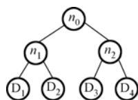
图 8.2 一棵哈希树
