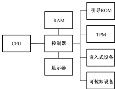
图 3.1 基于 TPM 的可信计算平台参考模型
