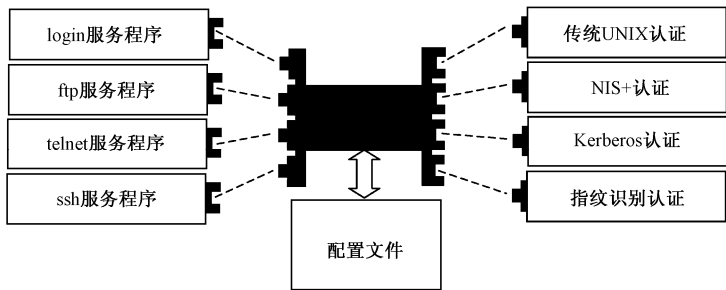
图 4.6 PAM 认证框架的基本思想
