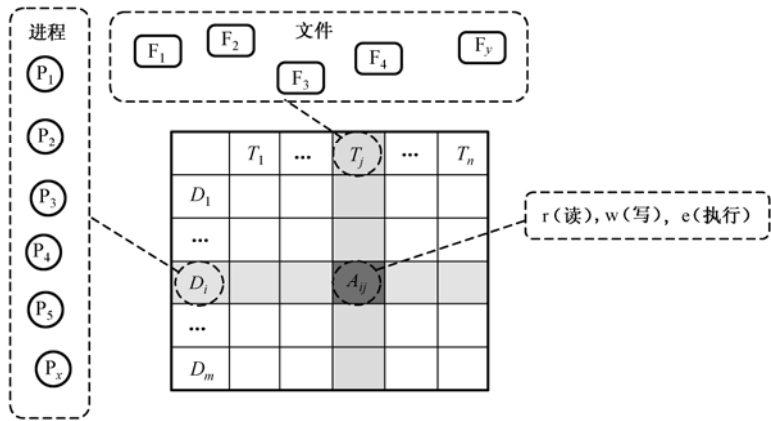
图 5.1 TE 模型的域定义表 (DDT)
