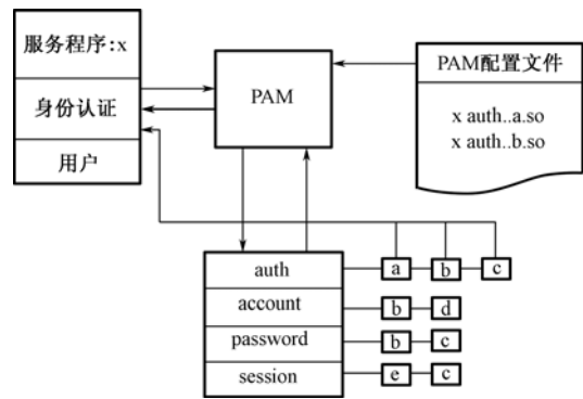
图 4.7 PAM 框架的基本结构和工作原理
