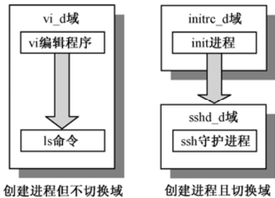
图 5.9 进程创建与域切换
