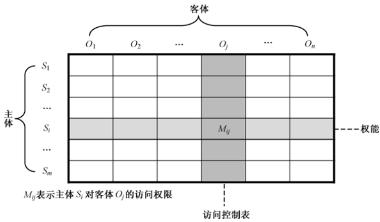
图 1.7 权能与访问控制表
