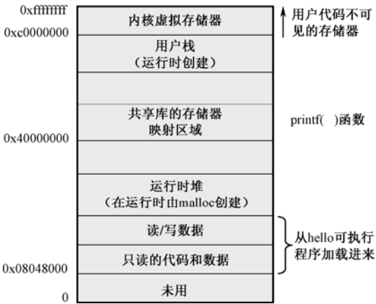
图 2.10 Linux 进程的虚拟地址空间
