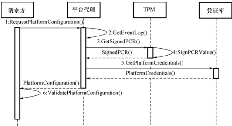
图 3.4 对外证明协议与消息交换
