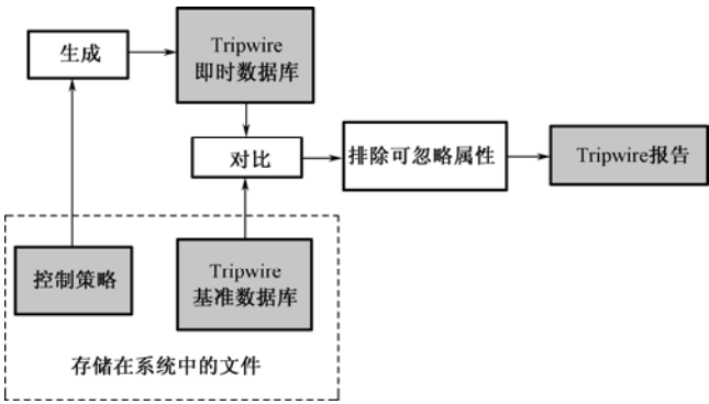
图 8.19 Tripwire 进行完整性检查的基本原理
