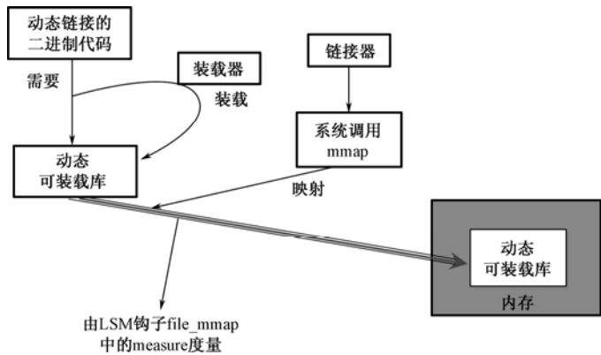
图 8.17 动态可装载库的装载和完整性度量
