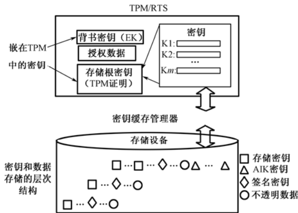
图 3.6 根密钥和真实身份密钥
