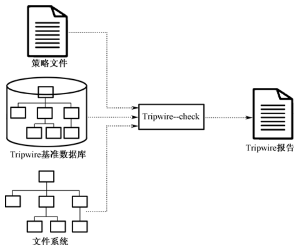
图 8.21 Tripwire 进行完整性检查
