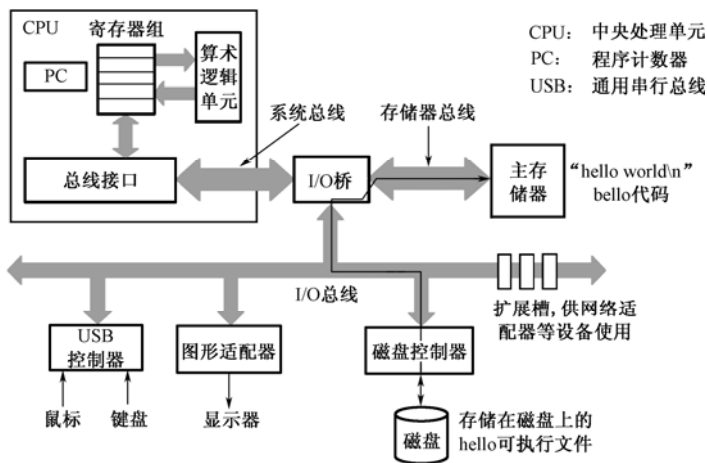
图 2.3 从磁盘加载可执行文件到主存
