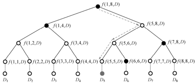
图 8.3 数据项 D_5 的完整性验证路径
