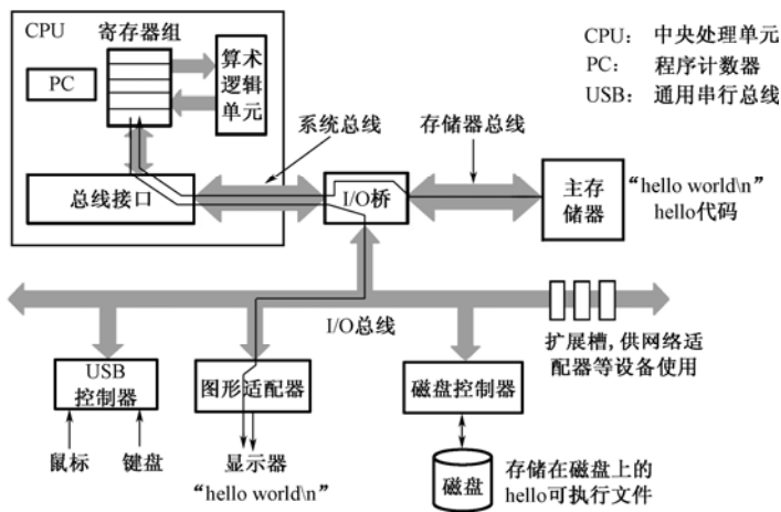
图 2.4 从存储器写输出串到显示器
