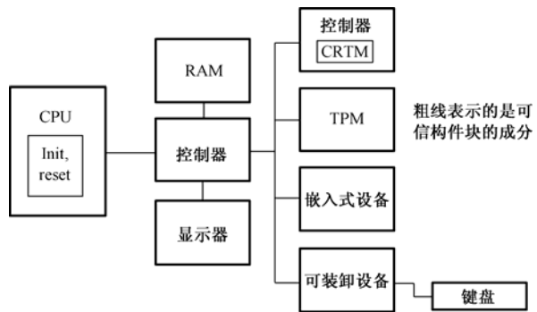
图 3.2 可信计算平台中的可信构件块
