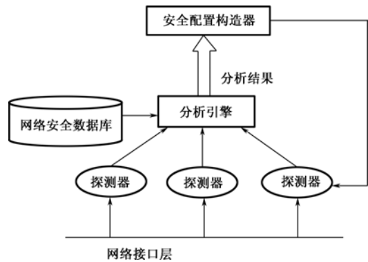
图 9.4 基于网络的 IDS 结构
