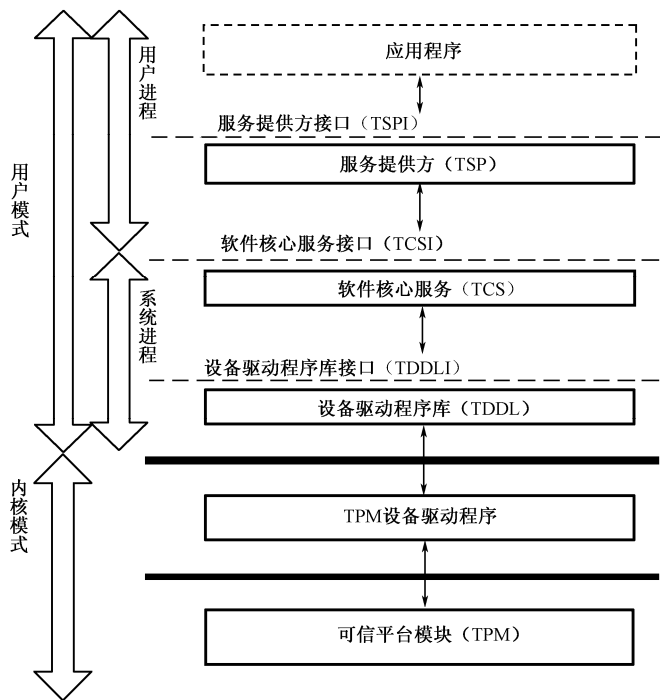
图 3.8 可信计算平台软件层次结构
