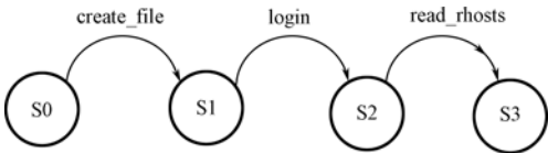
图 9.11 ftp-write 攻击状态转移图
