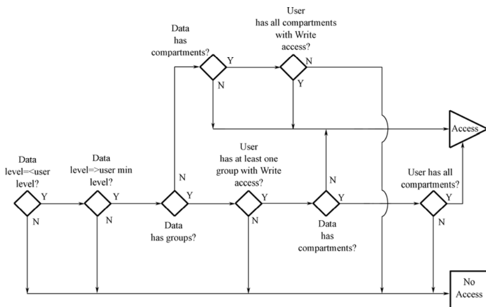
图 7.5 基于标签的写访问的判定过程
