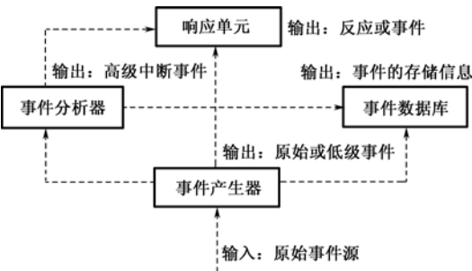
图 9.2 CIDF 基本模型
