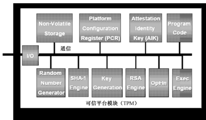
图 3.7 TPM 的逻辑结构及其构成组件
