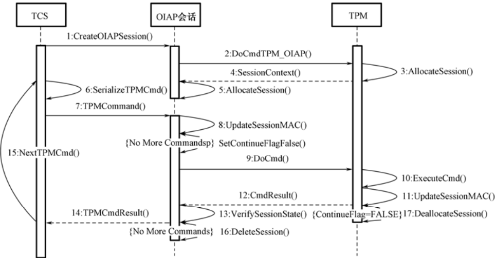
图 3.11 OIAP 的消息交换过程
