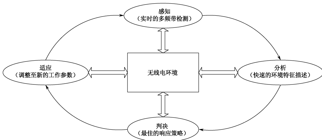
图 4-2 认知循环 [5]
