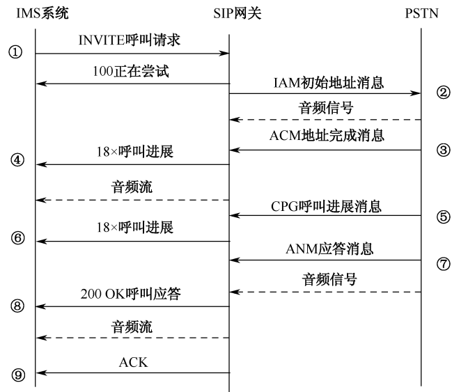
图 8-6 典型的信令网关协议转换流程
