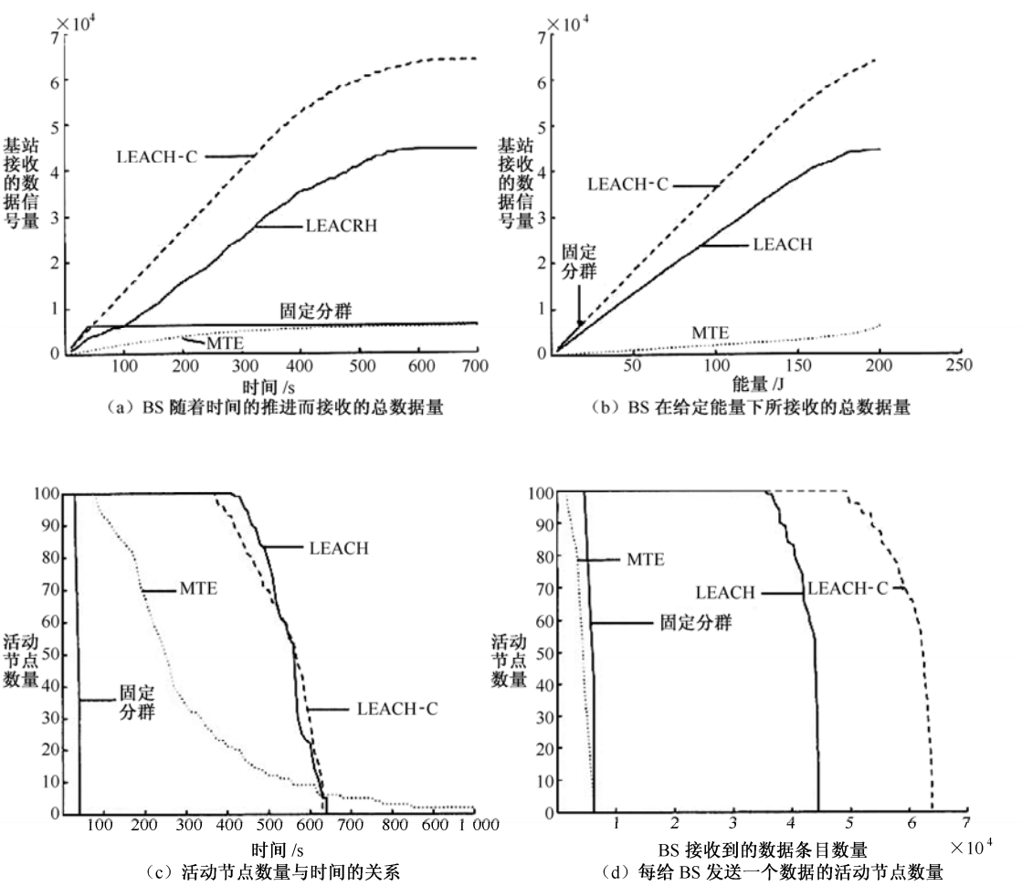
图 6-4 LEACH 的性能
