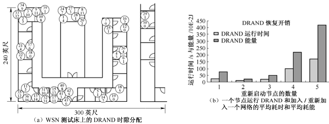
图 3-8 DRAND 的能耗
