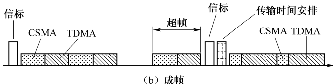
图 4-6 帧格式
