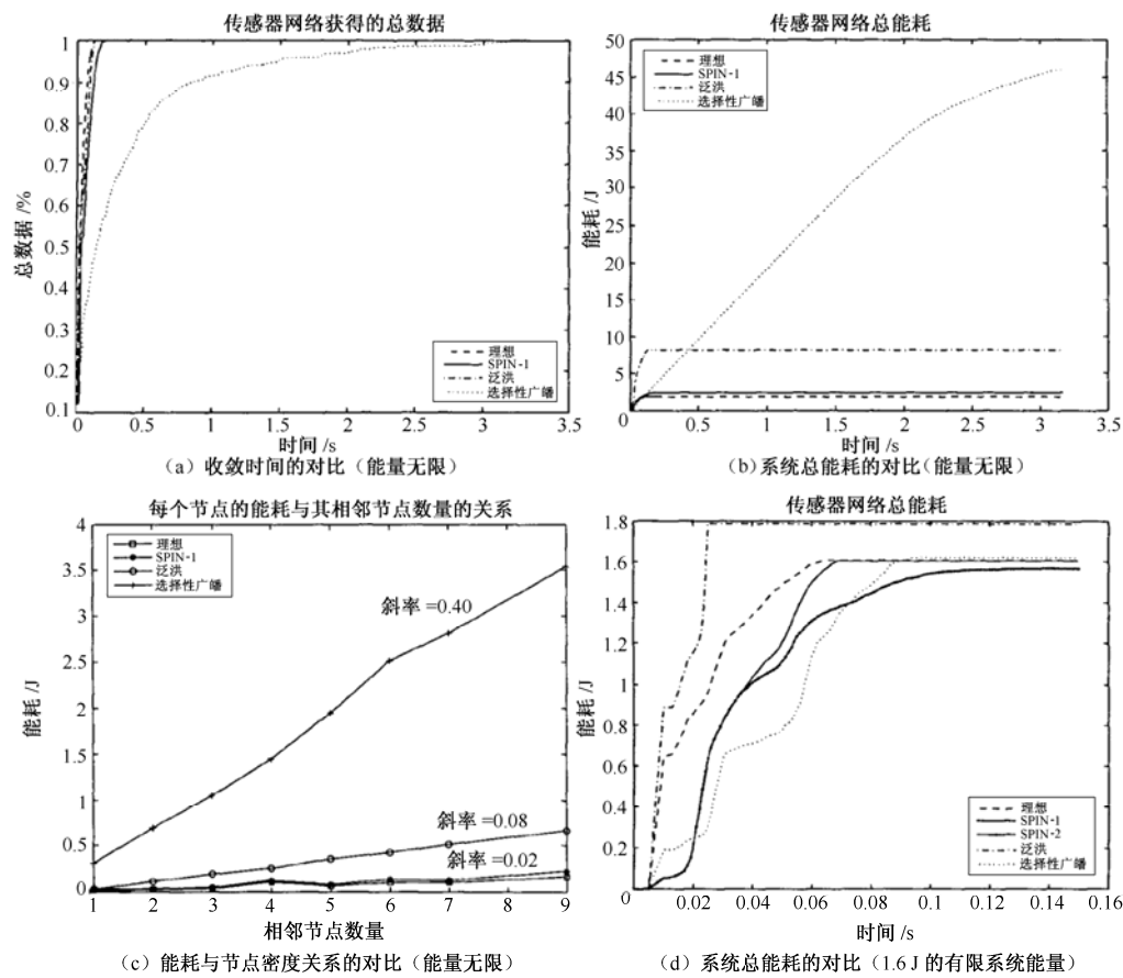
图 5-4 SPIN 的性能
