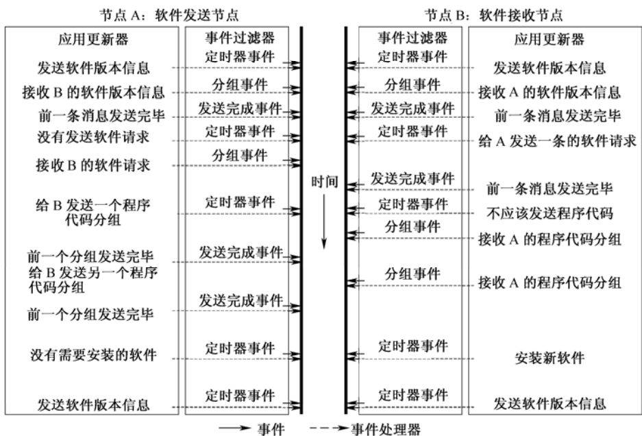
图 12-6 应用更新器
