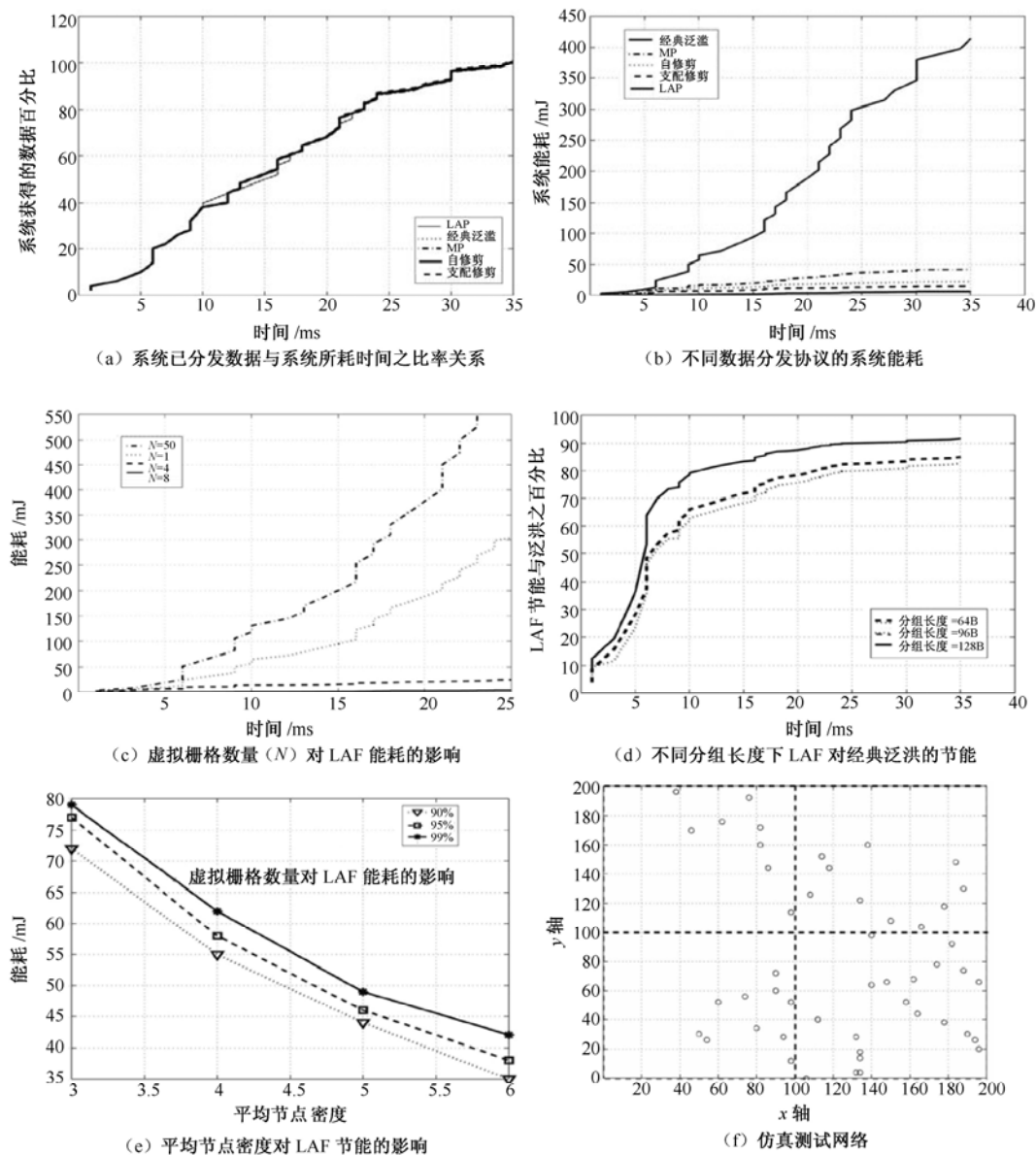
图 7-6 LAF 性能
