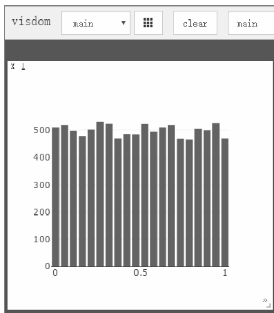
图 6.9 直方图
