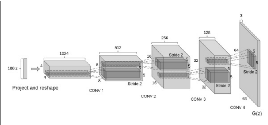
图 10.4 DCGAN 模型
