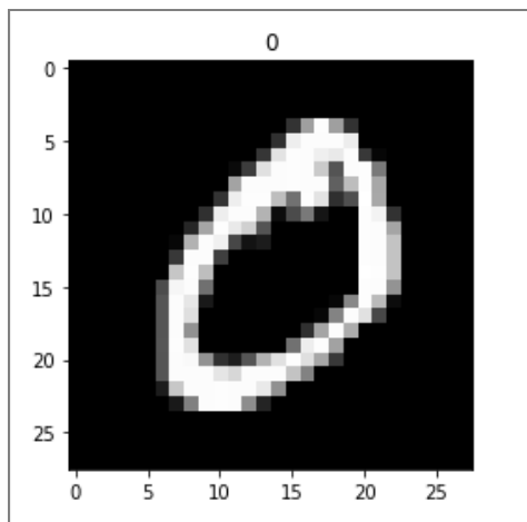
图 7.24 0 的手写照片
