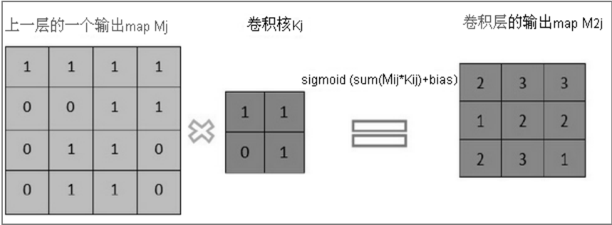
图 7.3 卷积运算
