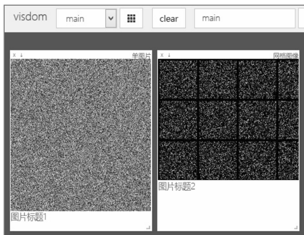
图 6.3 显示图片
