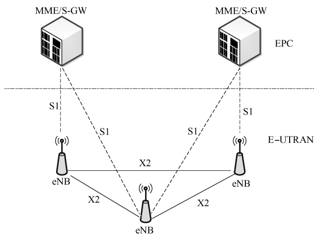
图 10-18 E-UTRAN 系统的总体架构
