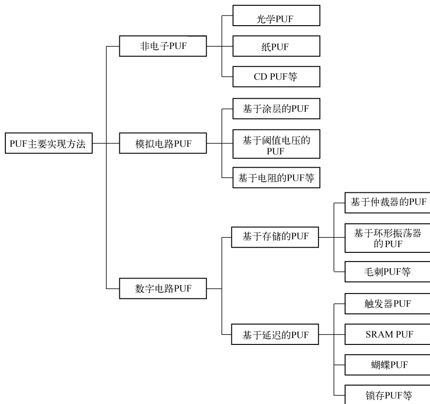
图 3-6 目前提出的主要物理不可克隆函数实现方法
