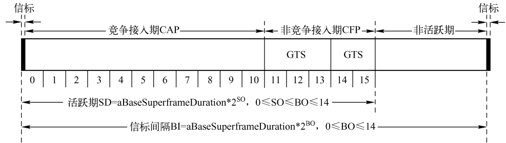
图 7-7 超帧结构
