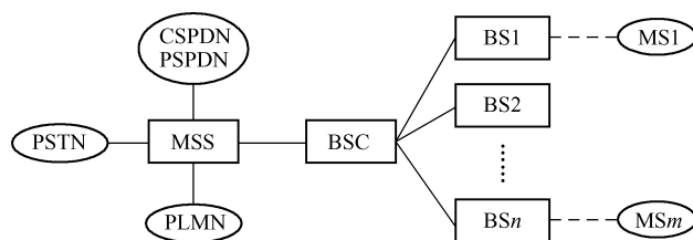
图 1-4 移动通信系统的基本组成
