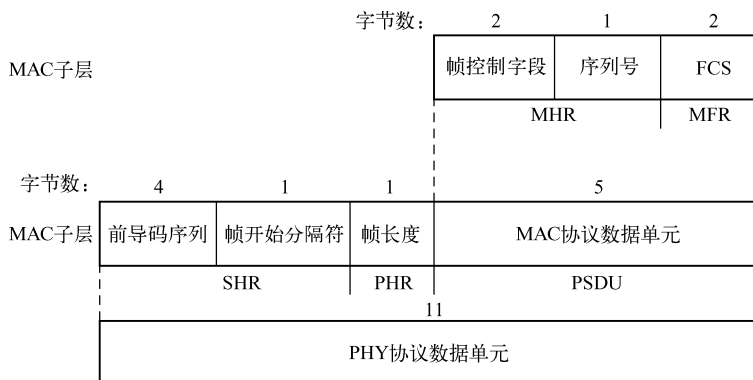
图 7-5 确认帧格式
