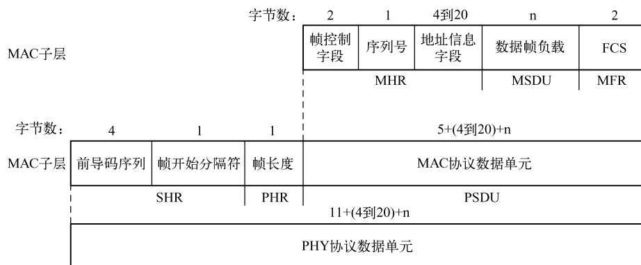
图 7-4 数据帧格式
