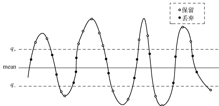
图 5-17 RSS 量化器
