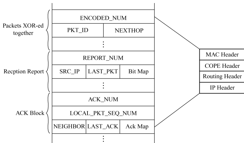
图 6-8 COPE 包头
