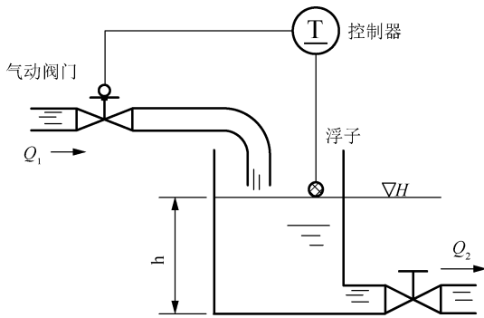
图 1-2 水箱液面自动控制
