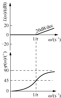
图 5-19 一阶微分环节伯德图
