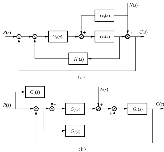
图 2-50 系统结构图
