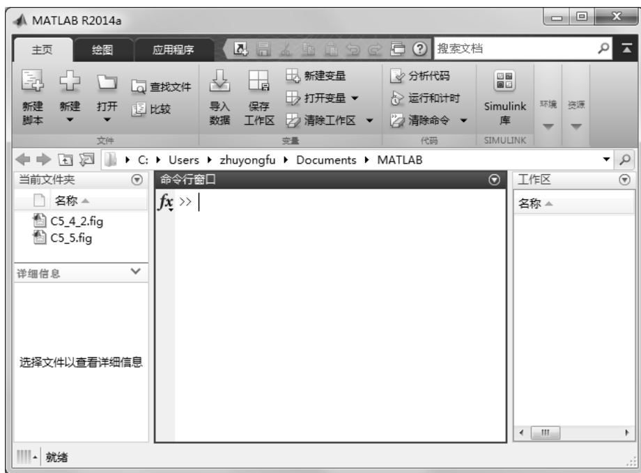
图 8-1 MATLAB 窗口
