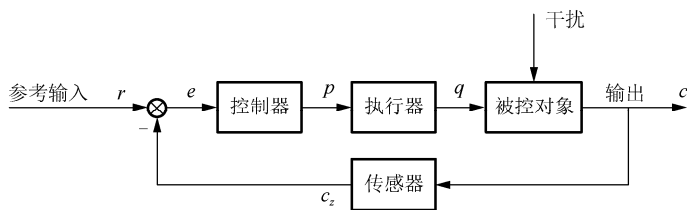
图 1-4 典型的自动控制系统框图
