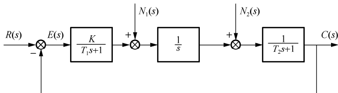
图 3-20 例 3-12 控制系统结构图
