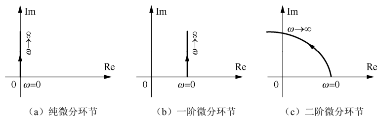
图 5-17 微分环节的奈氏图
