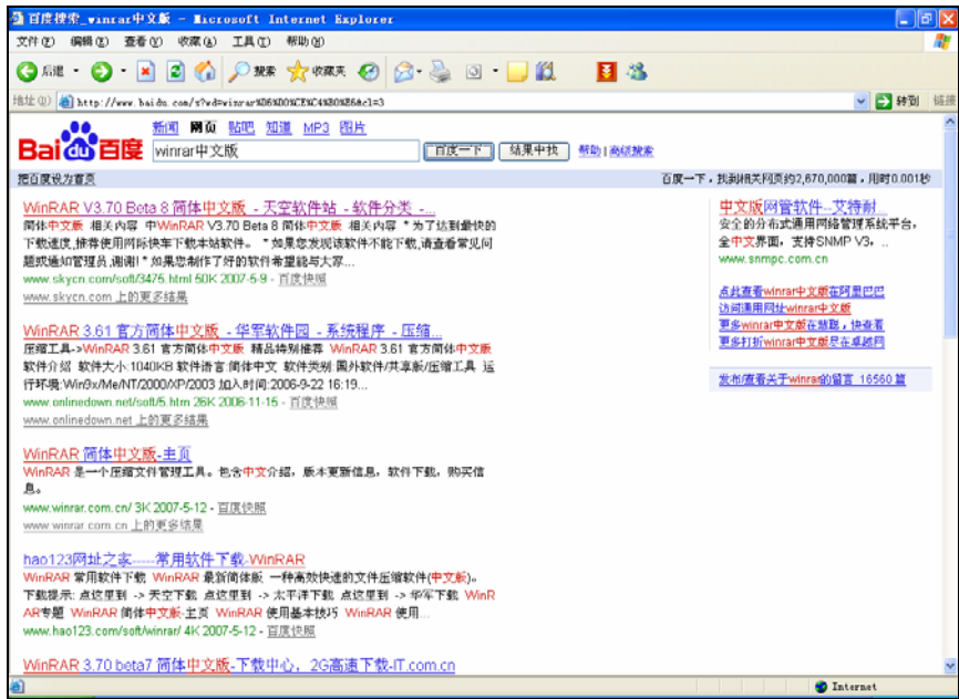
图 8-5 搜索 WinRAR
