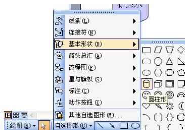
图 6-60 自选图形
