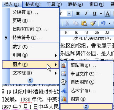
图 4-40 插入图片
