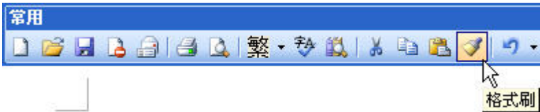
图 4-37 【常用】工具栏
