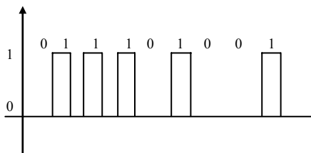
(a) 单极性归零码脉冲
