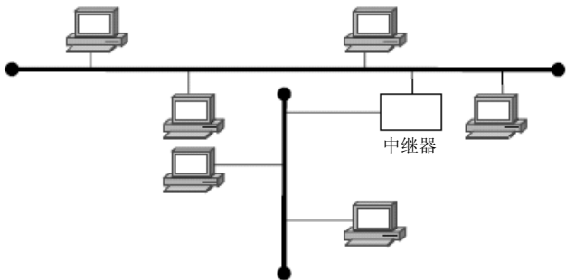
图 4-3 带有中继器的总线形拓扑
