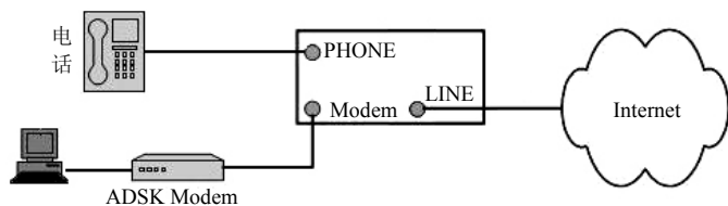
图 5-12 ADSL 接入 Internet
