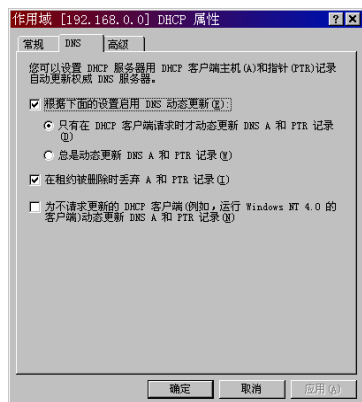
图 6-43 “DNS”选项卡
