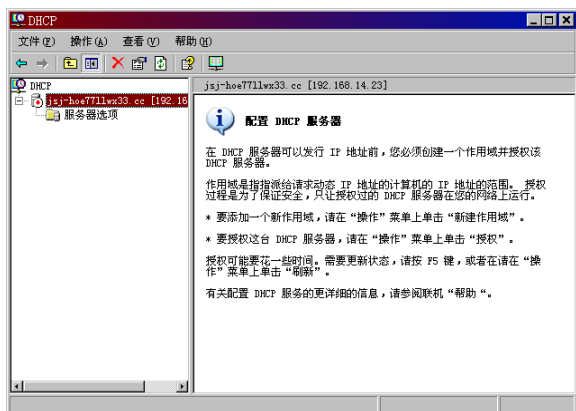
图 6-22 DHCP 控制台
