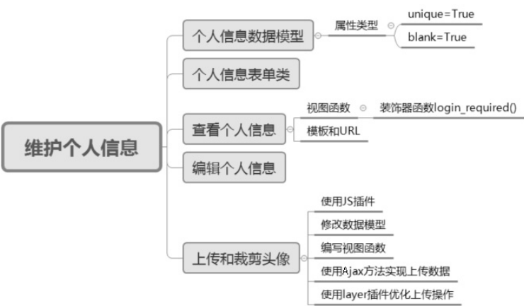
图 2-41 知识技能导图
