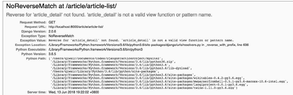
图 3-15 文章列表页报错
