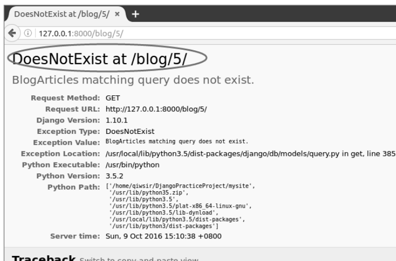
图 1-17 访问不存在的内容
