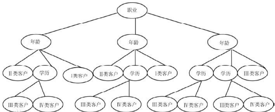
图 12-1 决策树算法的核心内容
