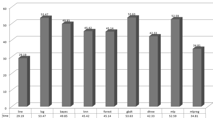
图 15-2 各种机器学习算法的准确度比较
