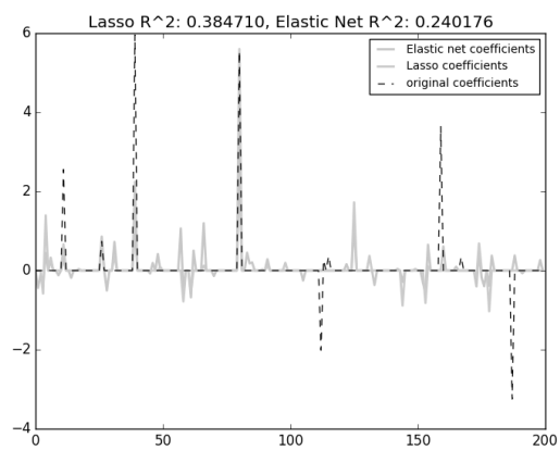
图 11-2 最小绝对值收缩和选择算法
