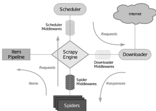
图 6-1 Scrapy 内部结构图
