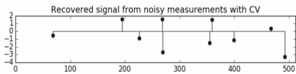
图 11-6 正交匹配追踪（OMP）算法
