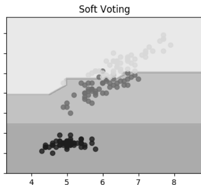
图 11-34 投票算法
