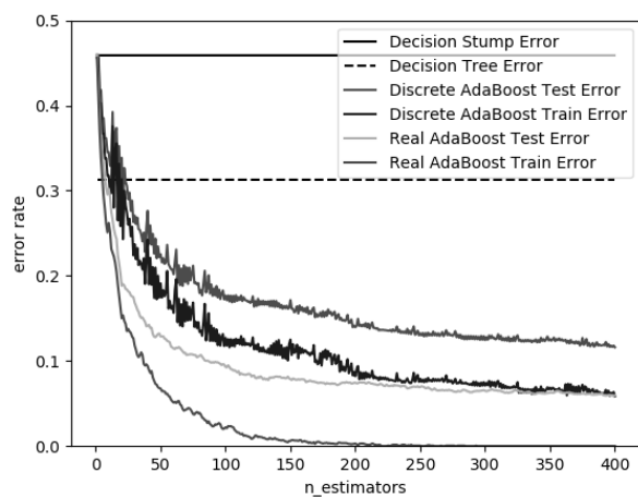
图 11-31 迭代算法
