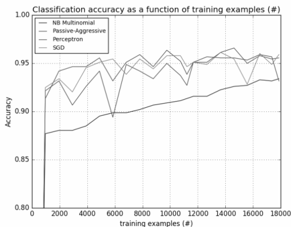
图 11-11 感知器算法
