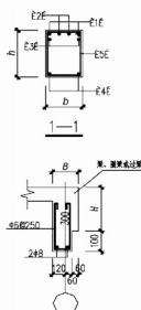
檐口线条大样图
