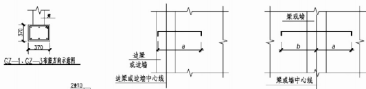
板顶支座钢筋长度示意图
