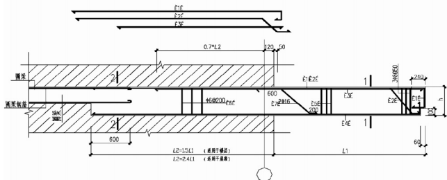
悬臂梁(XLx)配筋构造二
