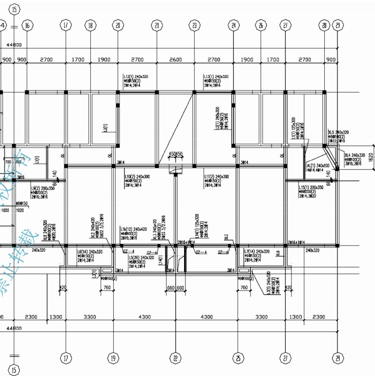
梁板配筋平面图
