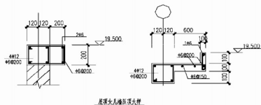
屋边女儿墙压顶大样
