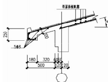
檐口大样图
