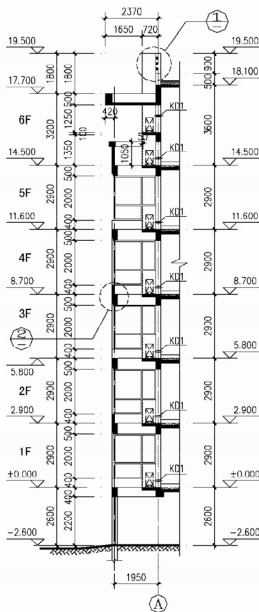
空调板位置剖面图
