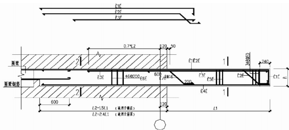
悬臂梁(XLx)配筋构造一
