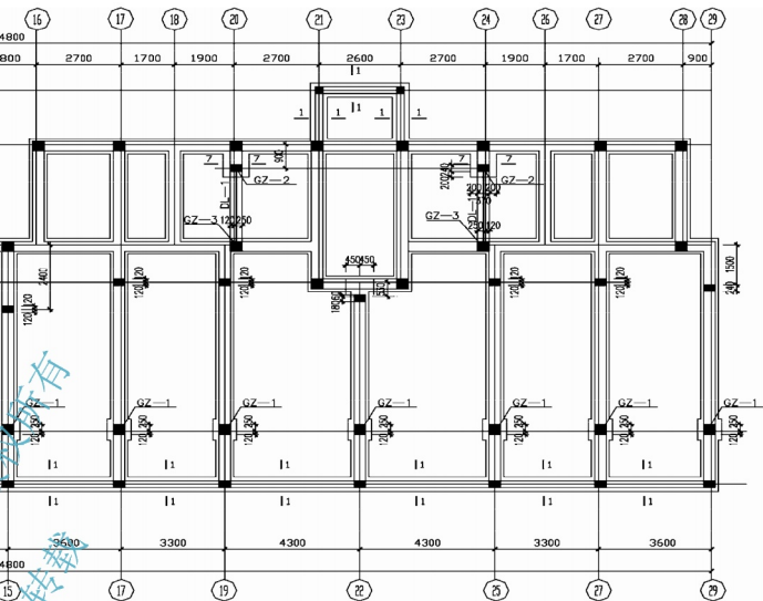
基础布置平面图
