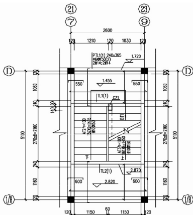
二层楼梯平面图
