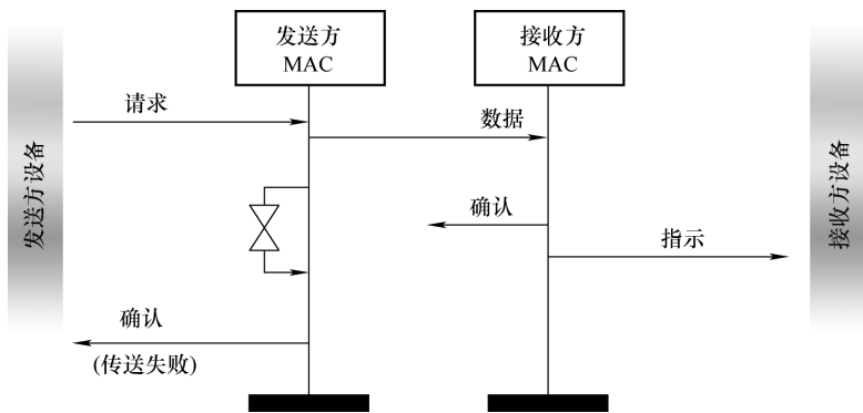
图 5-15 传输场景——丢失确认帧
