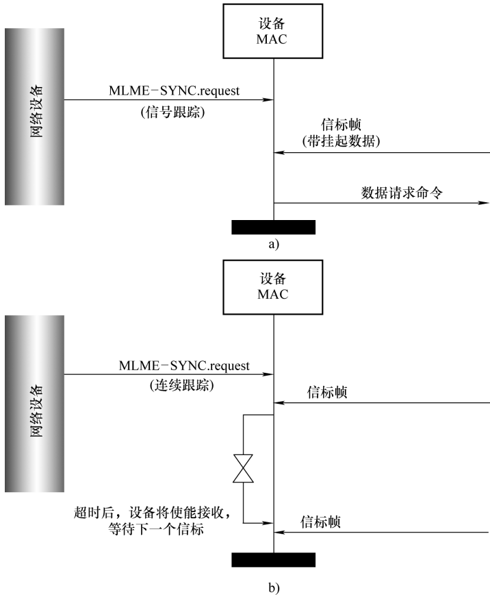
图 5-26 网络设备同步的报文序列图 a) 单次跟踪 b) 持续跟踪
