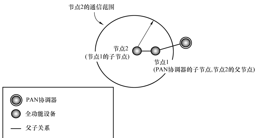
图 6-5 簇形网络形成过程
