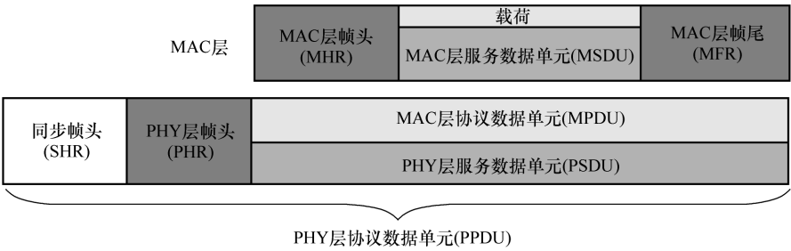
图 3-2 帧结构图
