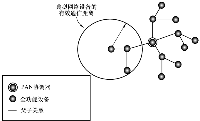
图 6-3 簇形网络
