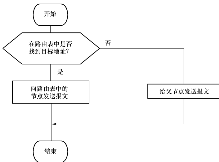
图 6-8 簇形网络的一种报文路由算法
