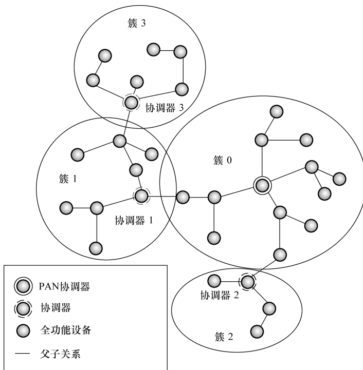
图 6-9 簇树形网络
