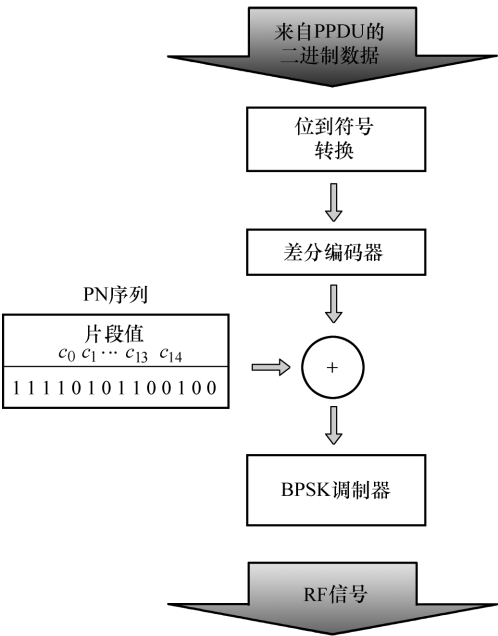
图 4-5 868/915MHz 频段的调制与扩展过程
