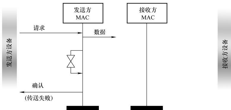
图 5-14 传输场景——丢失信息帧
