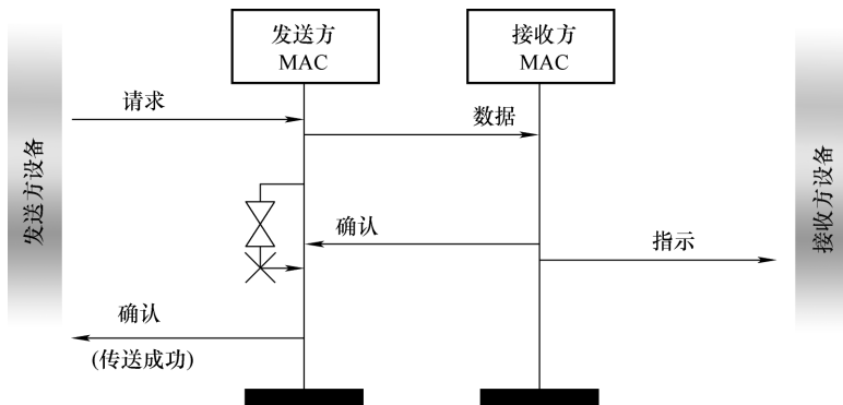
图 5-13 传输场景——数据成功传输
