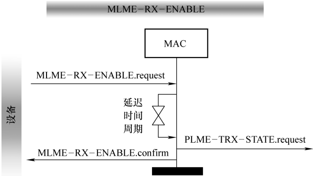
图 5-19 使能接收方的报文序列图
