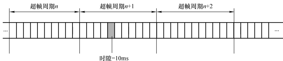
图 11-1 WirelessHART 超帧结构
