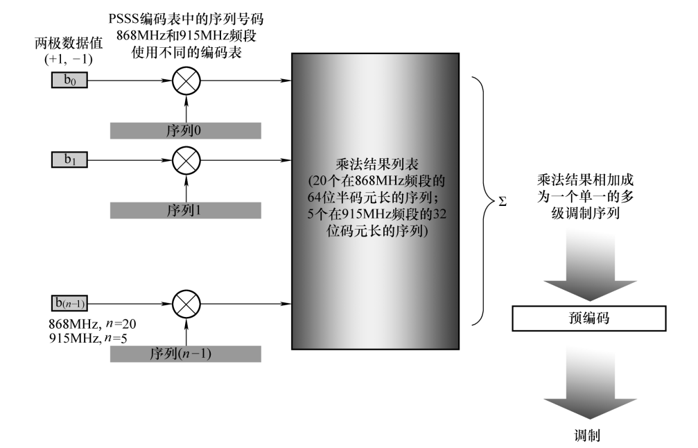
图 4-7 PSSS 模式物理层的符号到码元映射
