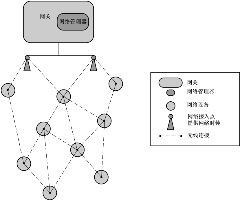
图 9-3 提供网络时钟的多个网络接入点
