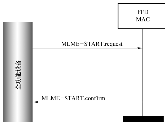
图 5-28 开始产生信标帧传输的报文序列图
