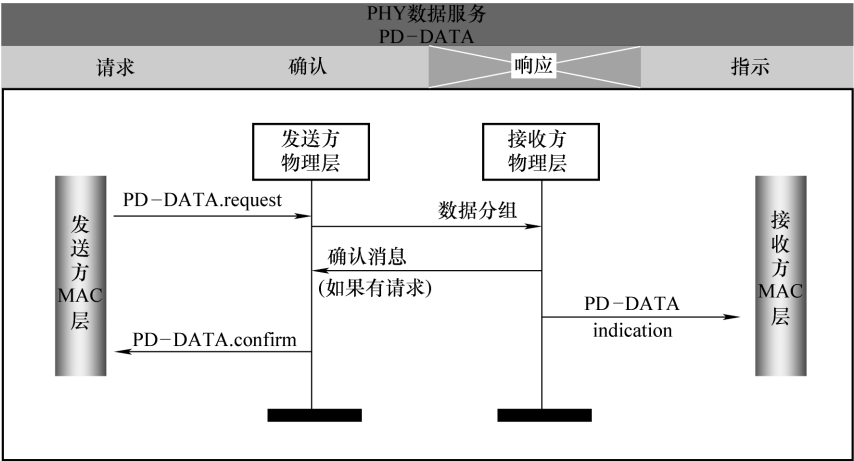
图 4-10 数据分组交换机制中的消息序列
