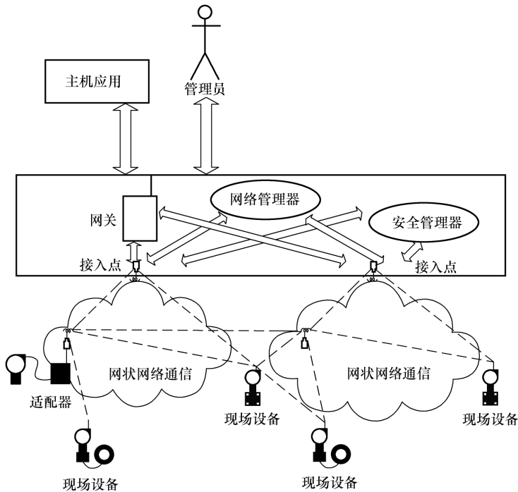
图 10-4 无线网络的网络结构图
