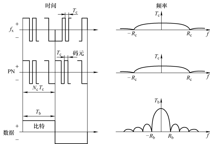
图 4-4 DSSS 解调（续）
