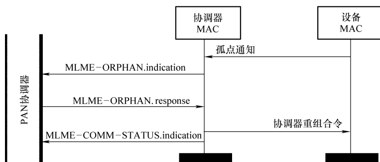
图 5-25 孤点通知机制的报文序列图
