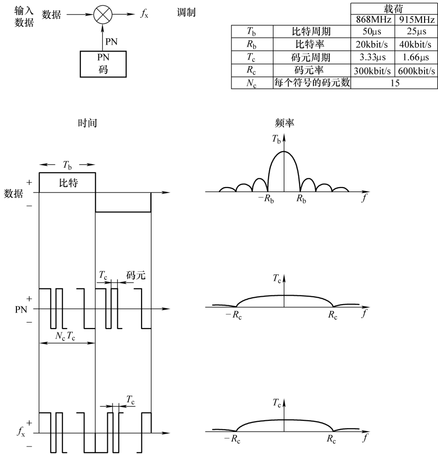
图 4-3 DSSS 调制
