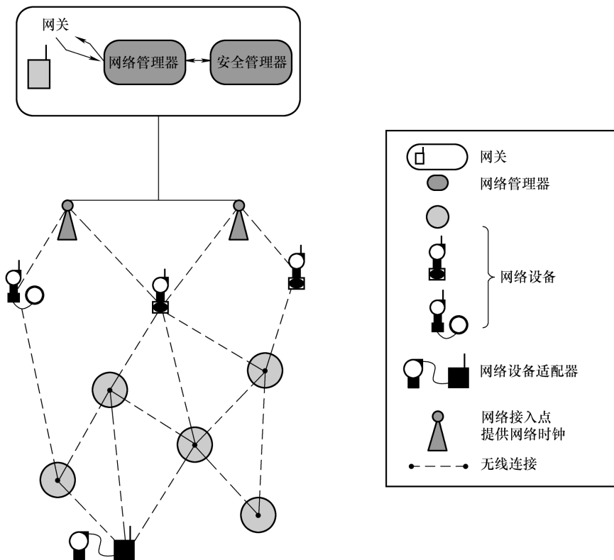
图 10-6 WirelessHART 网络中的网络管理器
