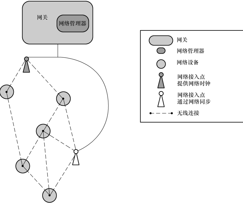
图 9-4 不提供网络时钟的多个网络接入点
