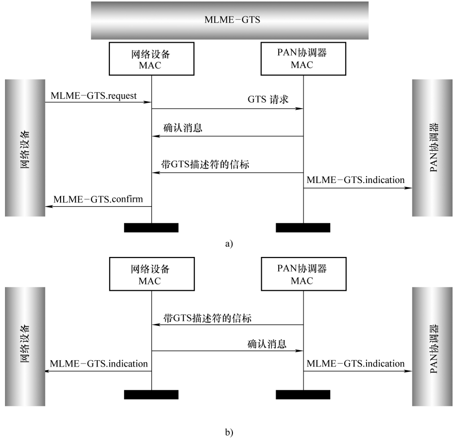
图 5-23 GTS 分配过程 a) 网络设备发起 b) PAN 协调器发起
