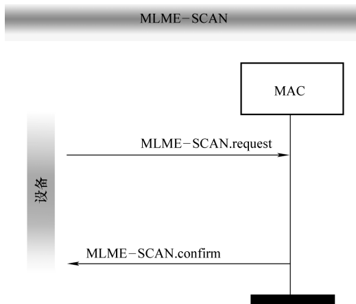
图 5-20 信道扫描机制中的报文序列图
