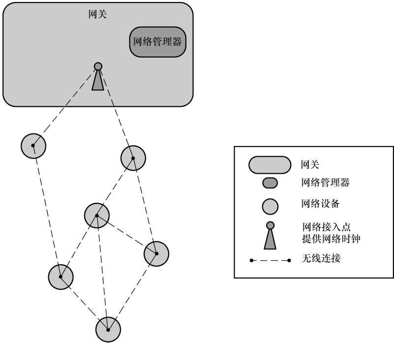
图 9-2 带时钟的单个网络接入点
