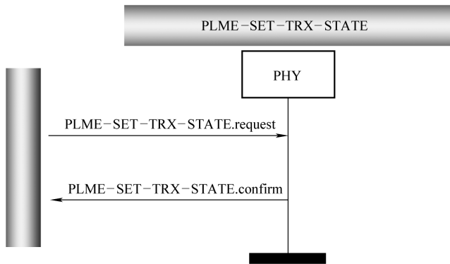
图 4-13 发送使能机制中的报文序列图
