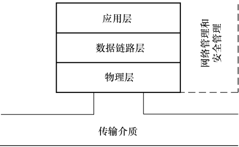
图 9-6 基本现场总线参考模型
