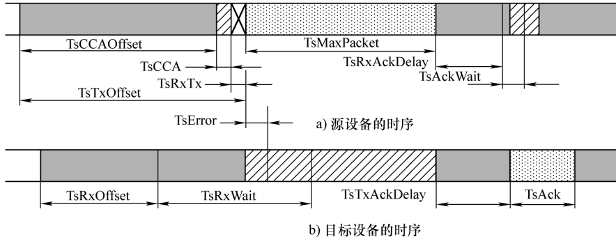
图 11-3 时隙的时序
