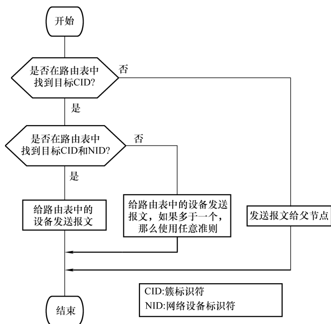
图6-10 一种簇树路由算法
