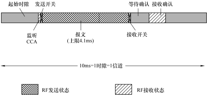
图 11-2 时隙结构总览图
