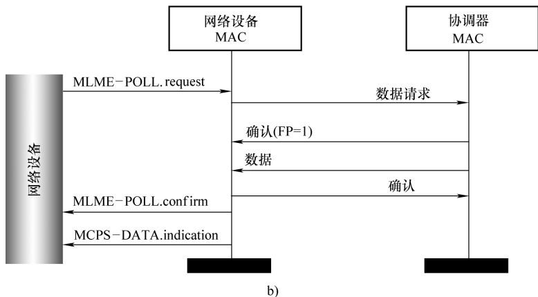
图 5-30 轮询协调器的报文序列图（续） b）有无待发数据
