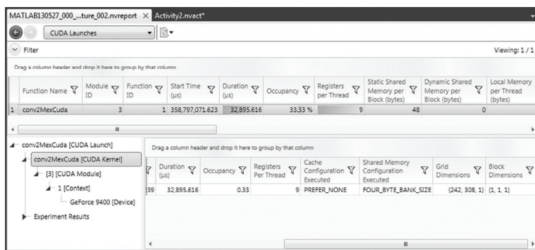
图 3.22 Nsight 窗口中 CUDA 内核函数和时间分析更多的细节信息
