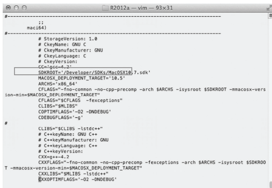
图 2.3 用于 Mac OS X SDK 选择的 mexopts.sh 文件
