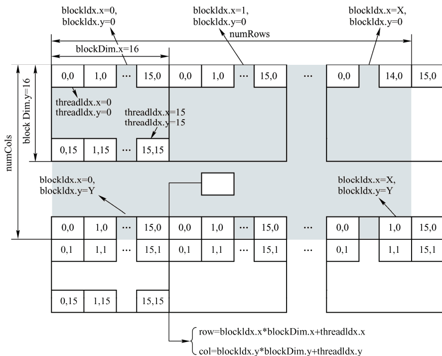
图 4.14 分配给图像的线程块和线程
