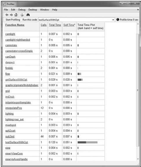
图 7.12 优化后的 MATLAB 代码时间分析
