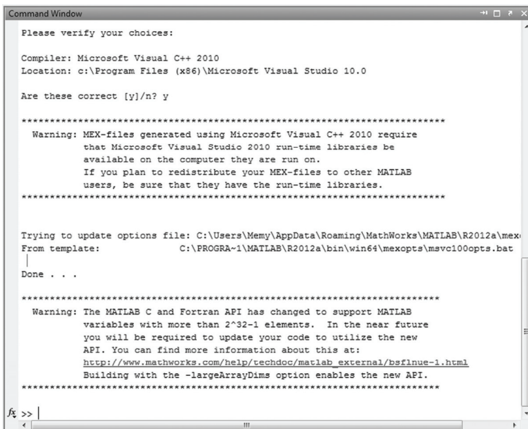
图 2.2 c-mex 配置中确认 C/C++编译器
