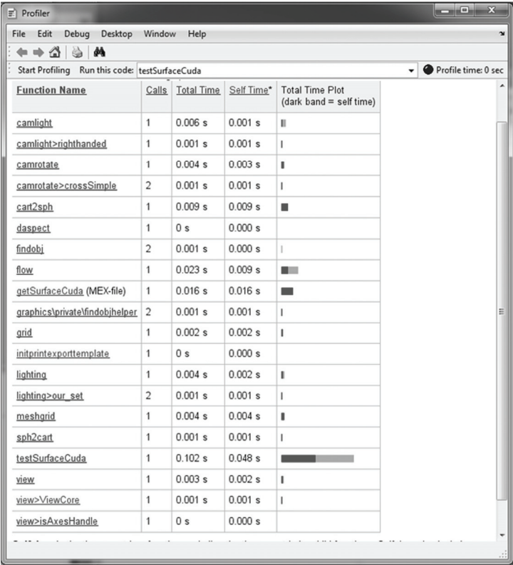
图 7.14 利用 GPU 的 c-mex 时间分析
