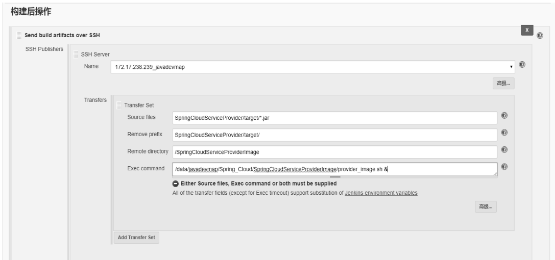
图 20-22 设置 Jenkins 推送目的地及脚本
