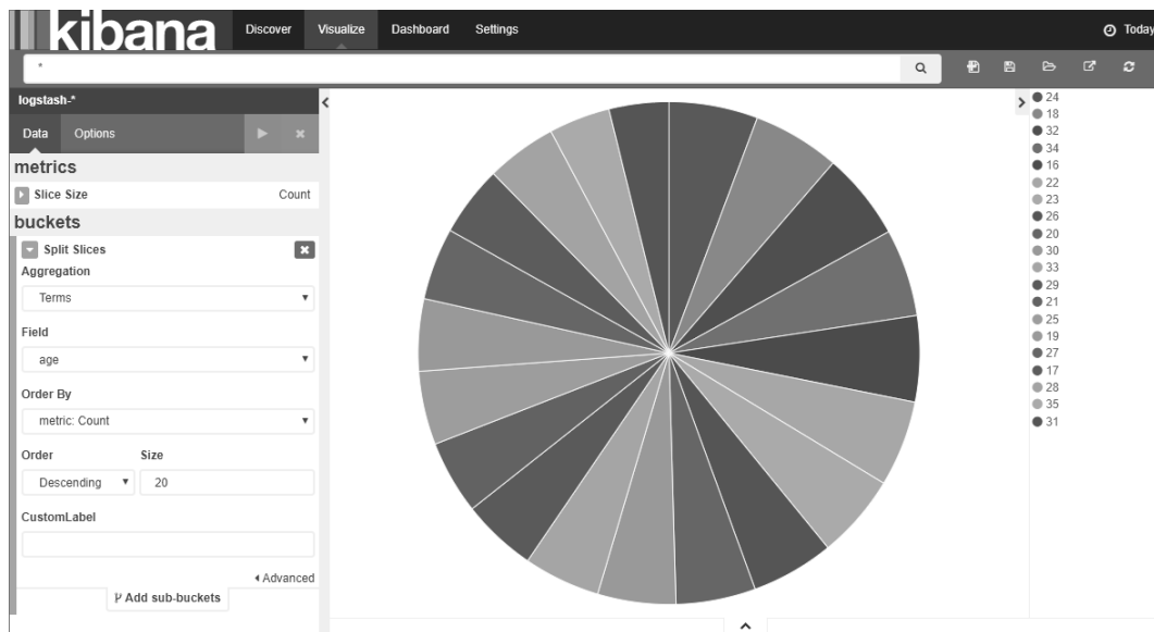
图 18-5 Kibana 饼图
