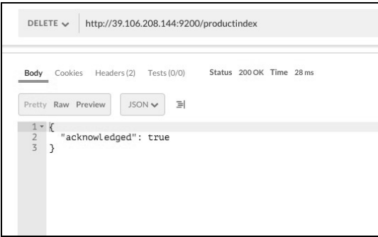
图 15-3 删除索引
