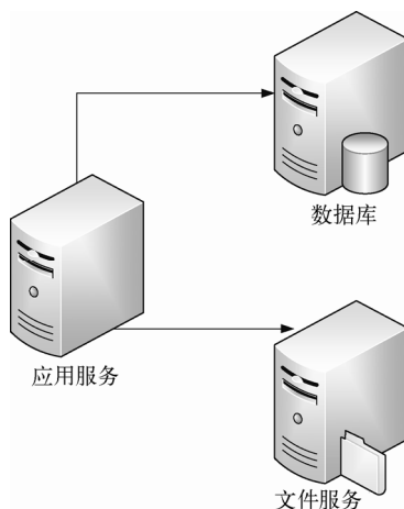
图 8-2 多台服务器
