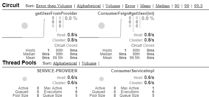
图 9-12 Hystrix 监控
