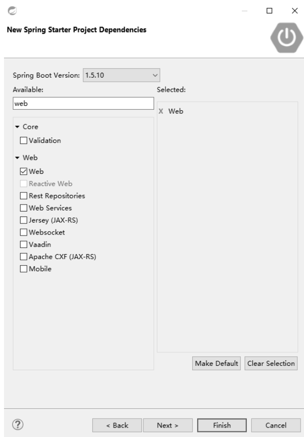
图 7-3 添加依赖
