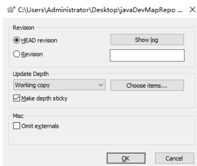
图 3-5 Svn 还原
