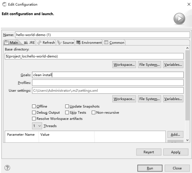
图 2-7 构建配置
