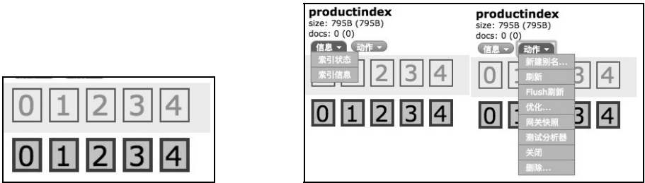
图 15-9 分片信息
