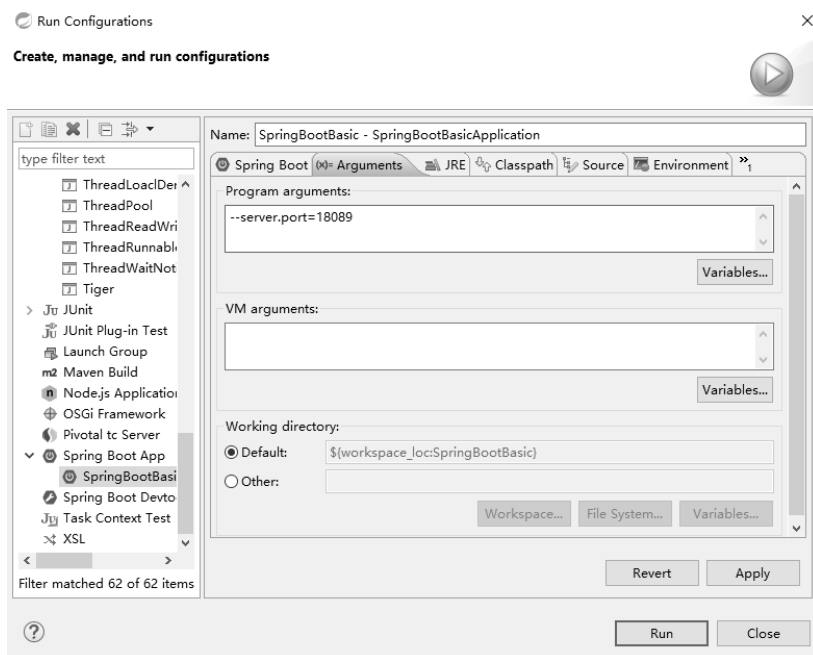
图 7-5 启动配置
