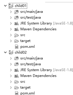
图 2-10 项目结构
