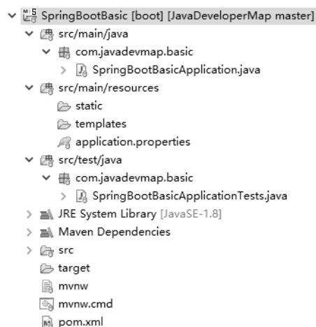
图 7-4 工程目录
