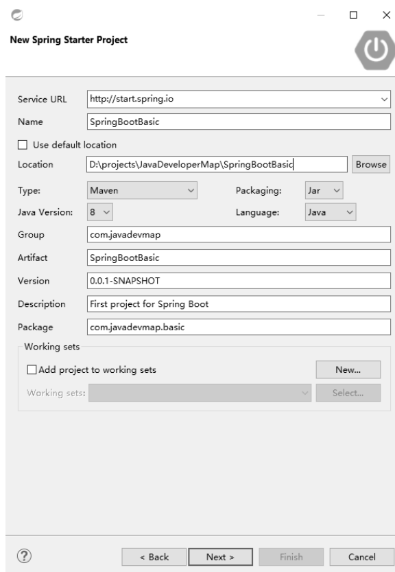
图 7-2 创建工程
