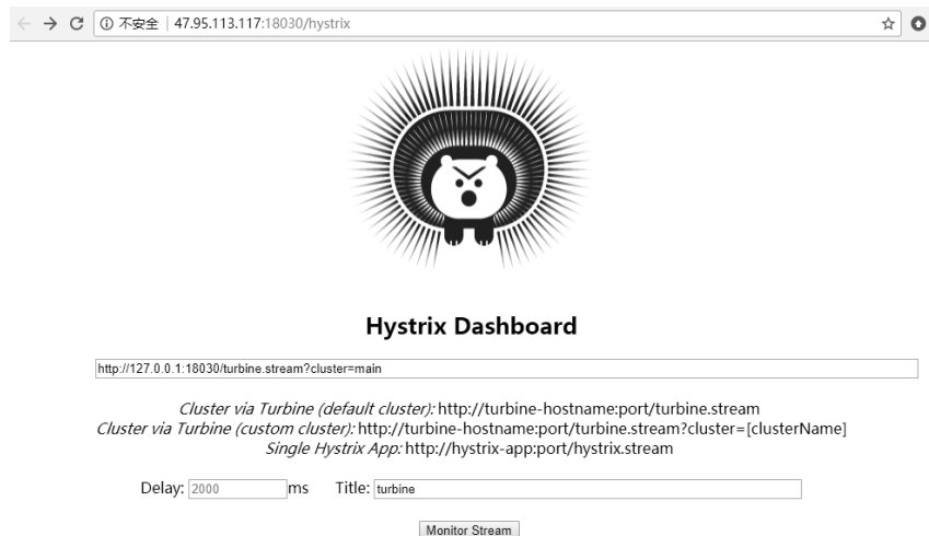
图 9-18 Turbine 配置
