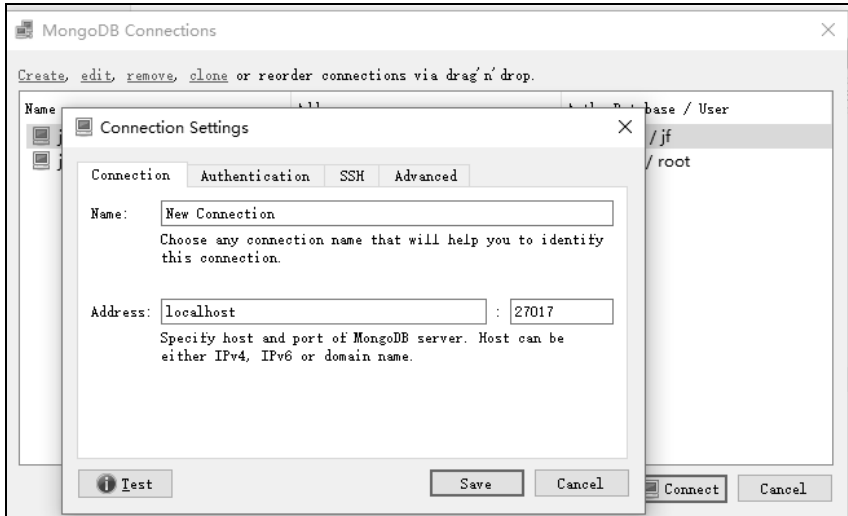
图 11-1 Robomongo 配置
