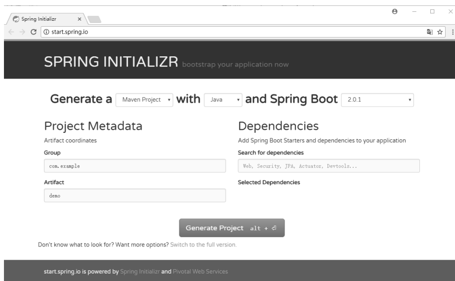
图 7-1 Initializr 页面
