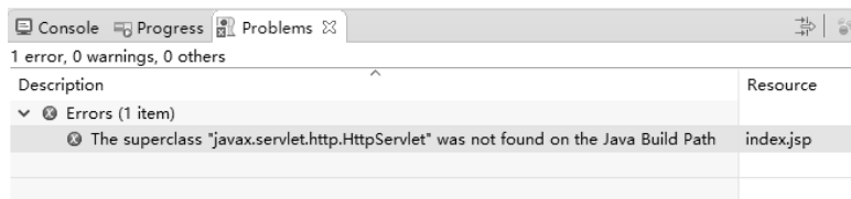
图 6-3 编译结果
