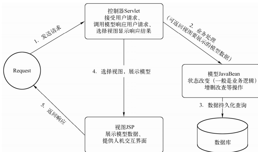
图 6-1 MVC 模块
