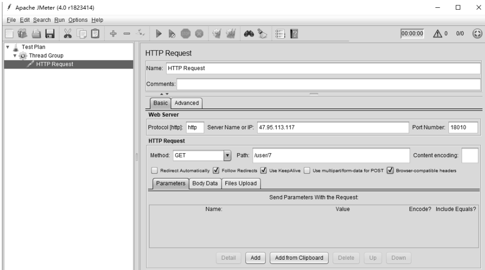
图 21-6 添加采样器
