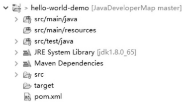
图 2-5 项目结构
