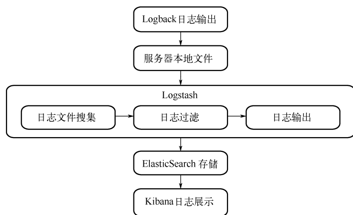
图 18-1 日志搜集
