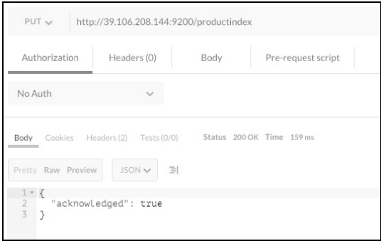
图 15-2 创建索引
