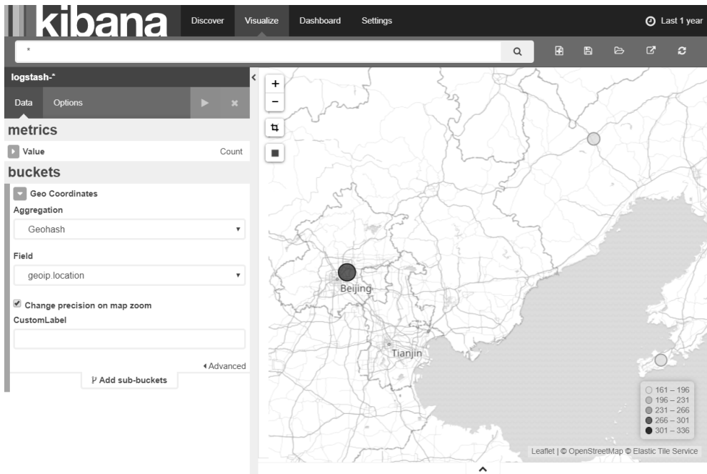
图 18-7 Kibana 地图
