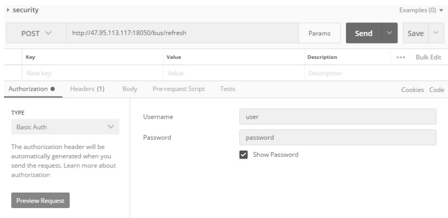
图 9-35 带安全组件的配置刷新
