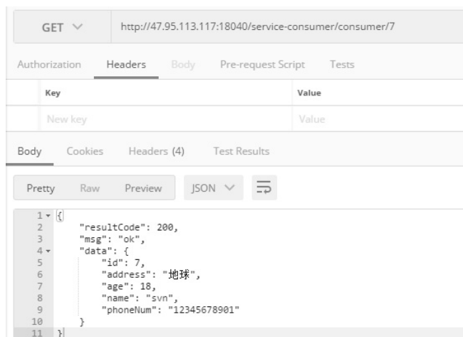
图 9-23 带路由的服务请求
