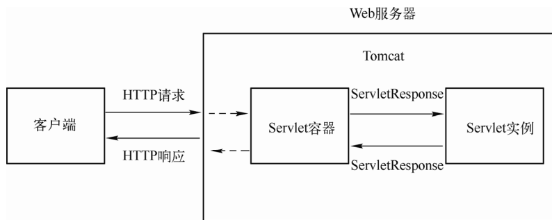
图 6-2 Servlet 与 Tomcat 的关系
