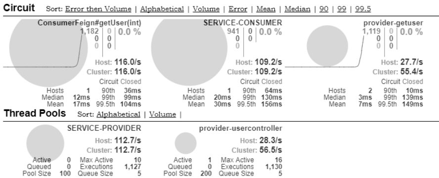
图 9-30 带 Zuul 服务的监控页面
