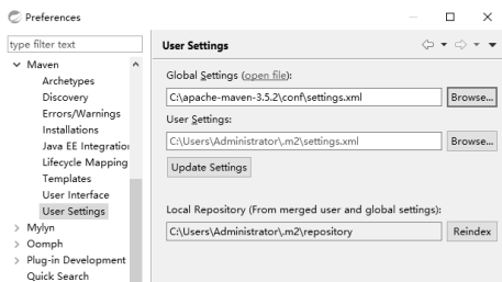
图 2-3 Maven 设置
