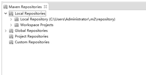
图 2-4 Maven 仓库
