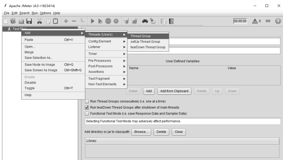
图 21-5 新建线程组
