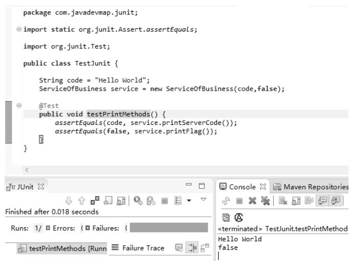
图 1-2 测试结果
