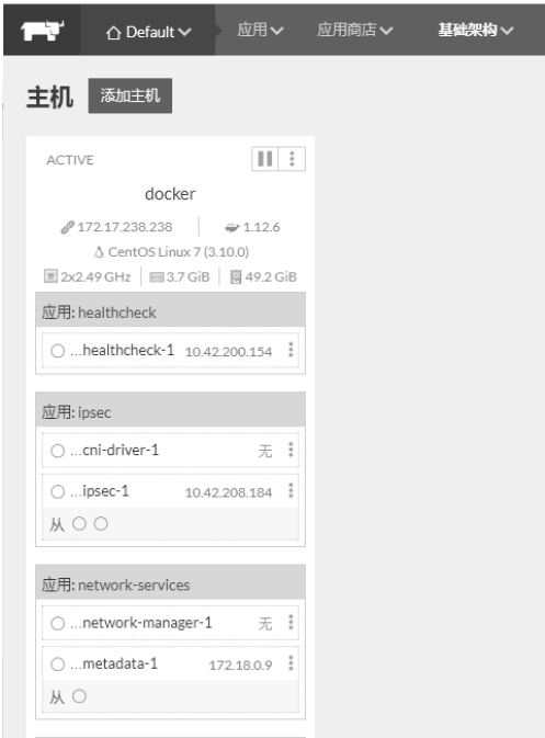
图 20-27 主机实例
