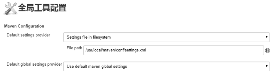
图 20-7 配置 Maven
