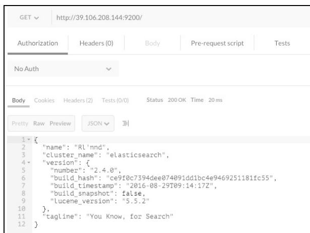
图 15-1 Elasticsearch 信息
