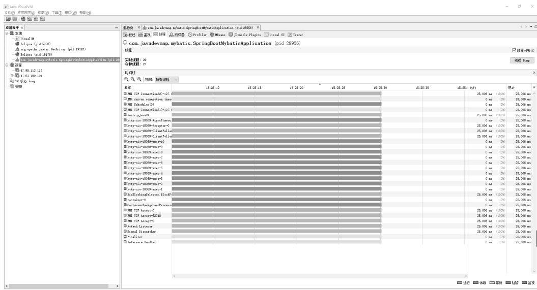
图 21-10 线程监控
