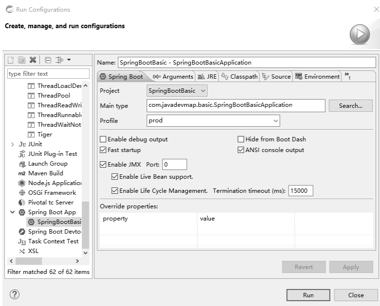
图 7-6 多环境选择
