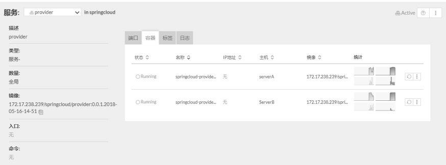
图 20-37 服务启动
