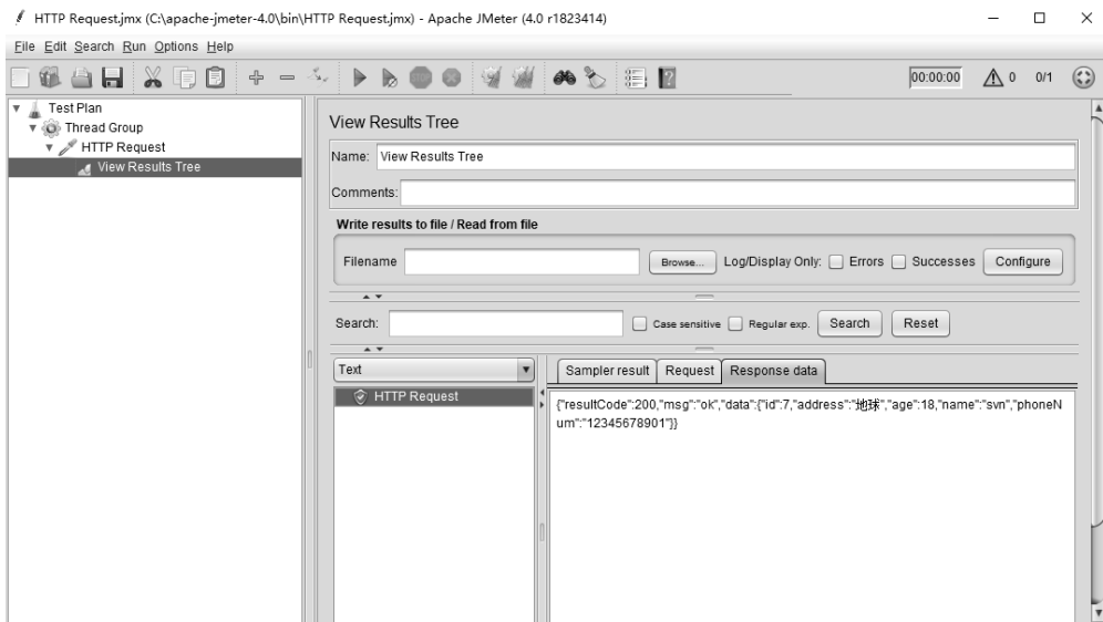
图 21-7 添加监听器
