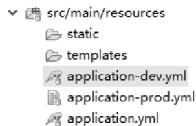
图 7-7 多配置文件
