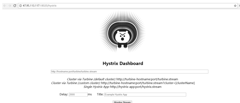
图 9-8 Hystrix 页面
