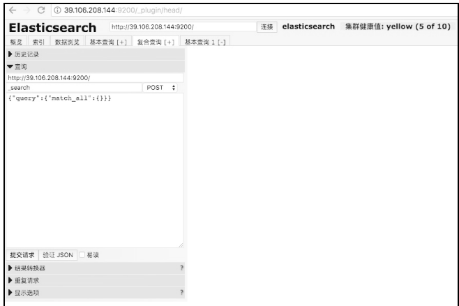
图 15-14 复合查询
