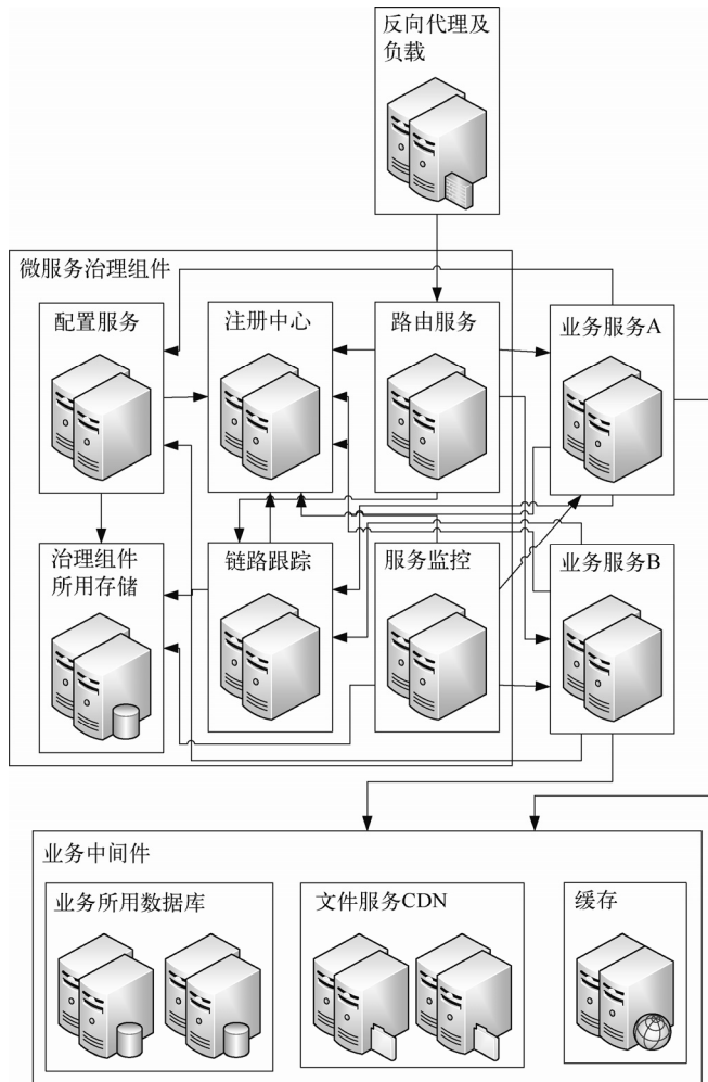
图 8-5 微服务集群
