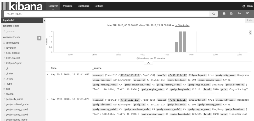
图 18-4 Kibana 搜索
