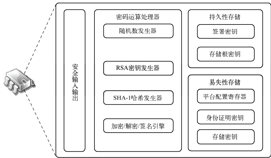
图 12-2 TPM 架构
