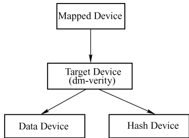
图 13-3 dm-verity 架构
