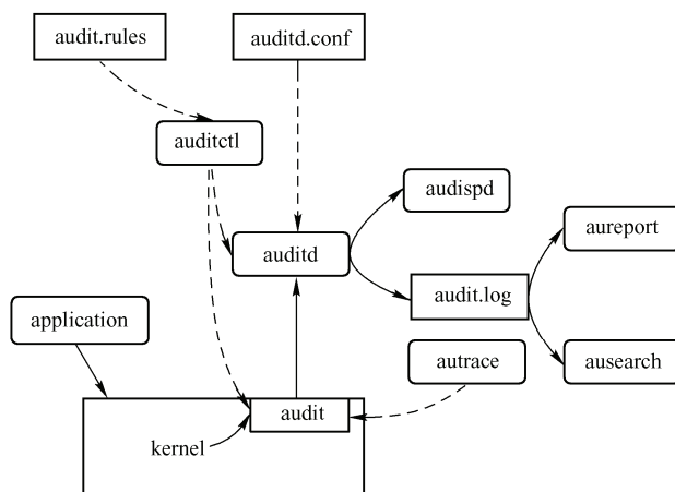
图 14-1 audit 架构
