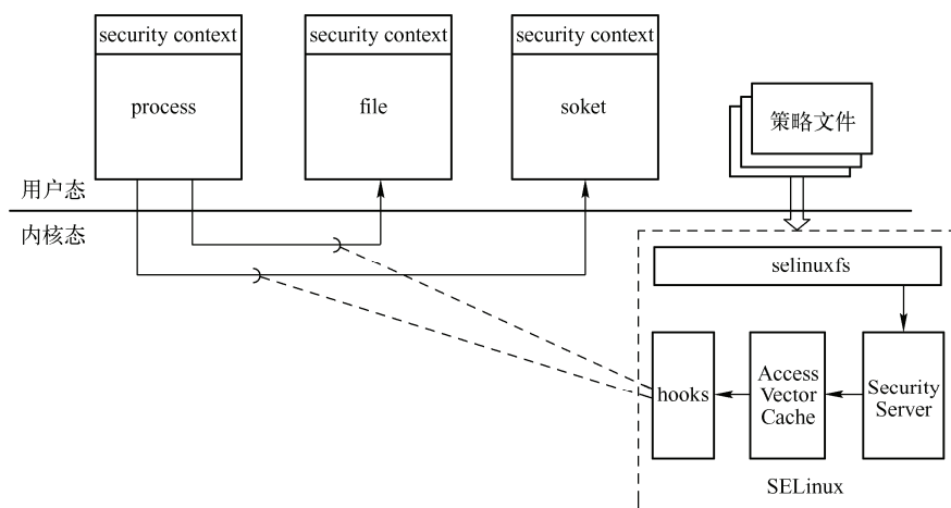
图 7-3 SELinux 架构
